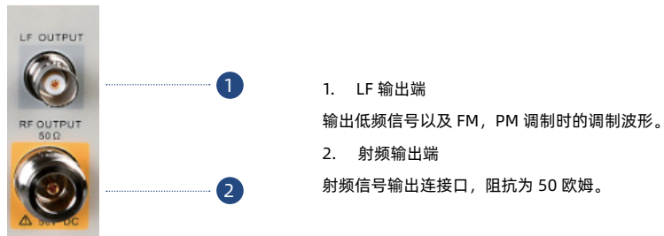
图 1- 6 前面板连接器
