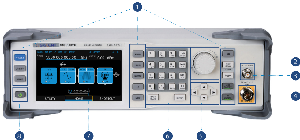
图 1- 4 前面板
