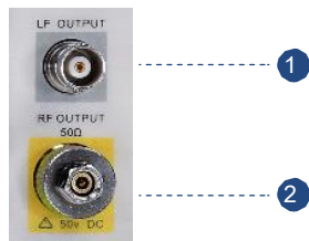
图 1-6 前面板连接器
