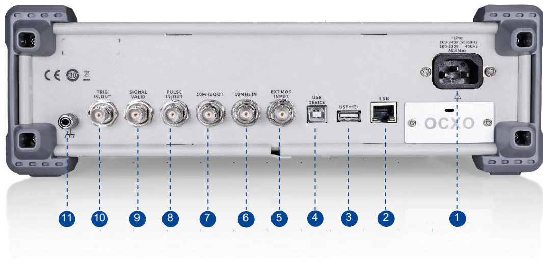
图 1-7 后面板
