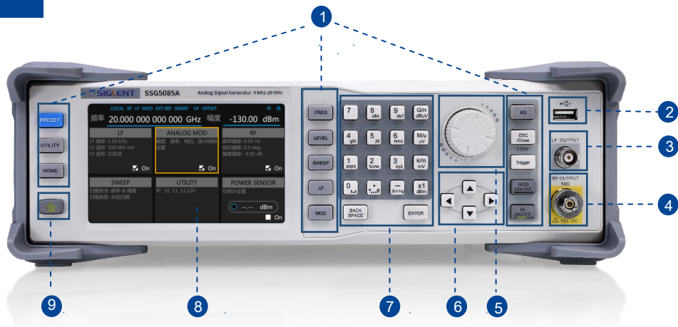
图 1-4 前面板
