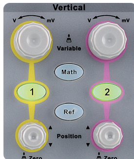
2通道垂直控制界面
