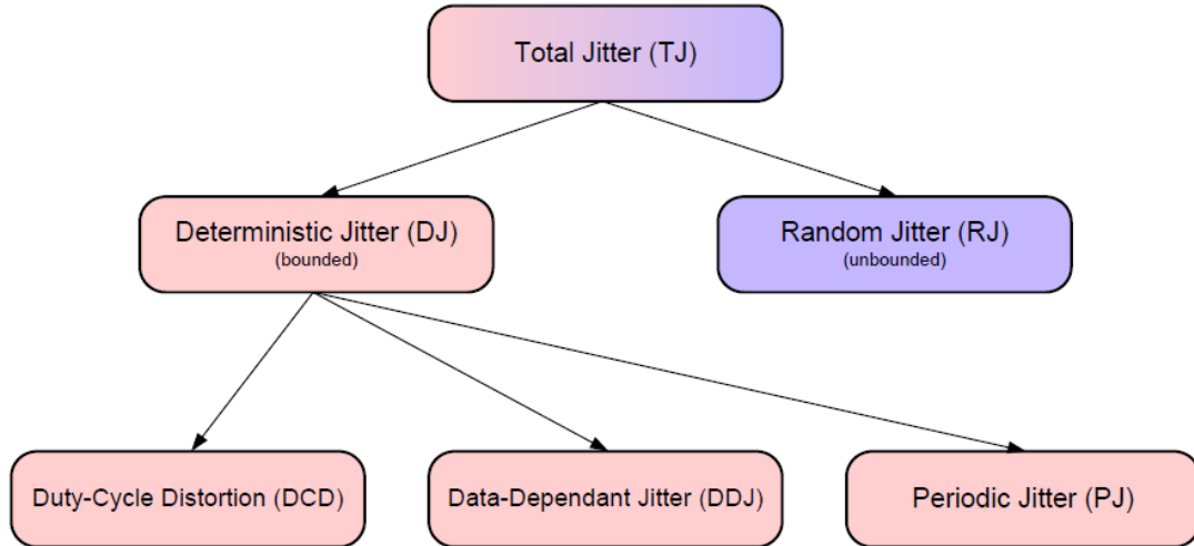
图 29.1 抖动的分解
