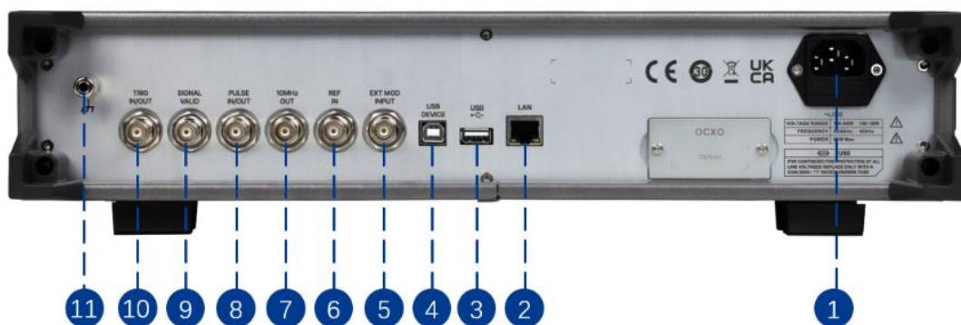
图 1-9 后面板
