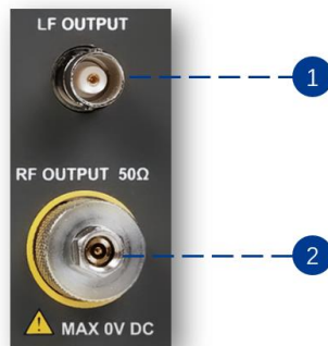
图 1-8 前面板连接器
