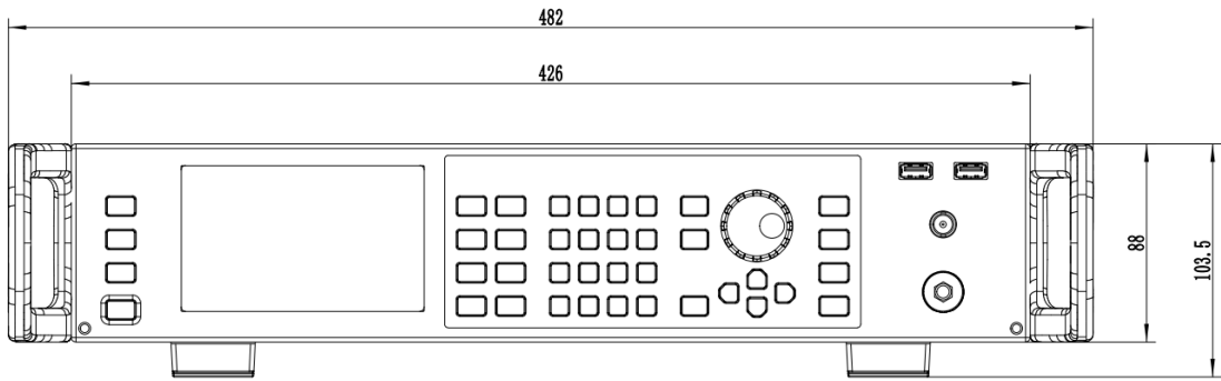
图 1-1 正视图
