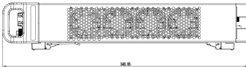
图 1-3 侧视图
