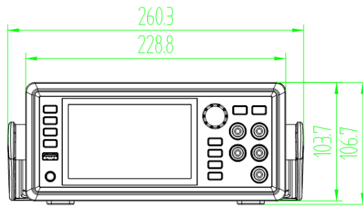
正视图
