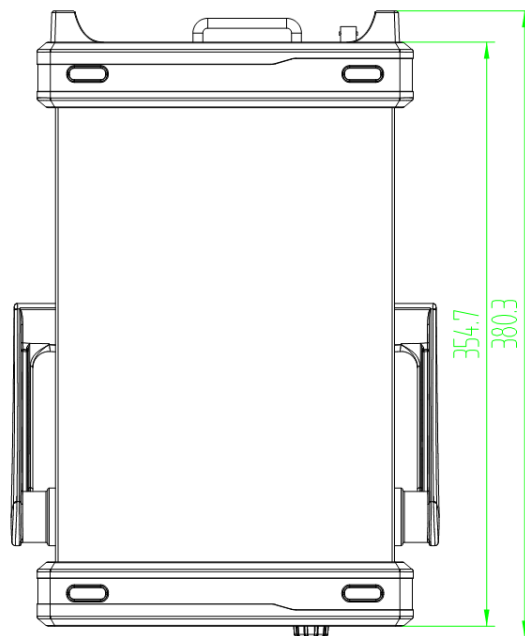
俯视图
