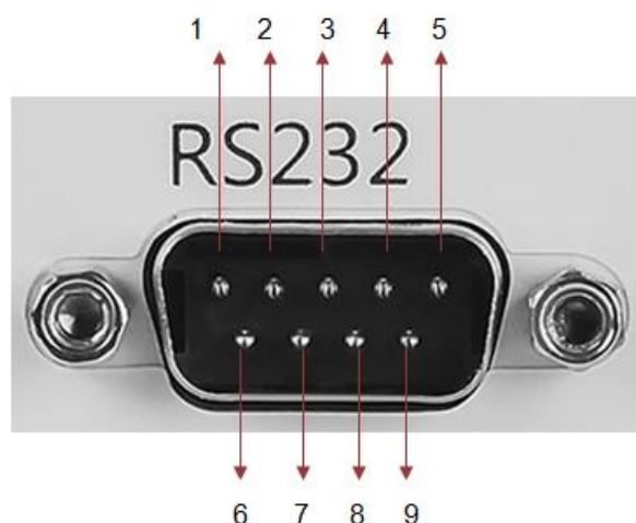
图 3-5 RS232 接口
