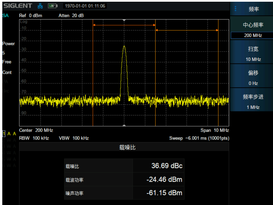
图 3-13 载噪比
