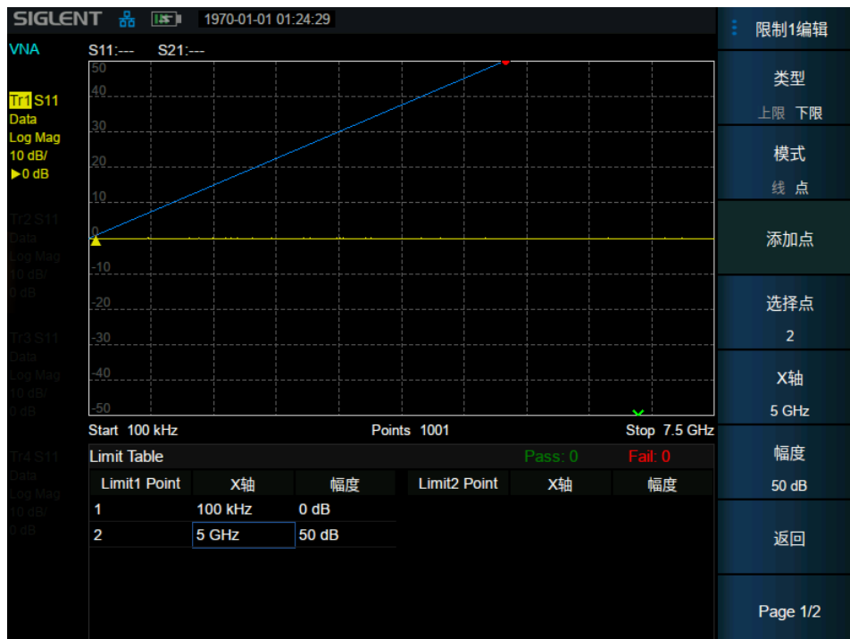
图 10-3 限制编辑
