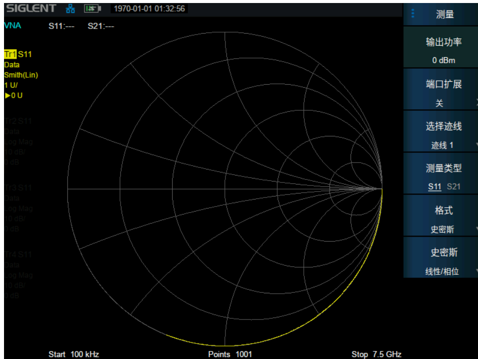
图 10-4 史密斯图
