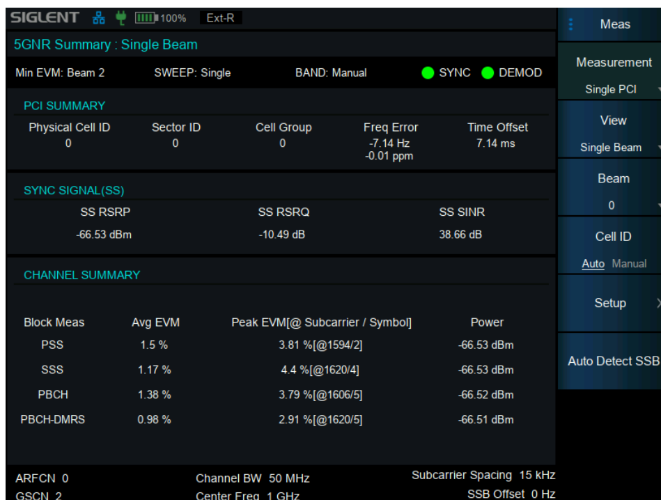
图 5-1 单波束视图
