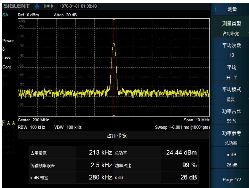
图 3-9 占用带宽
