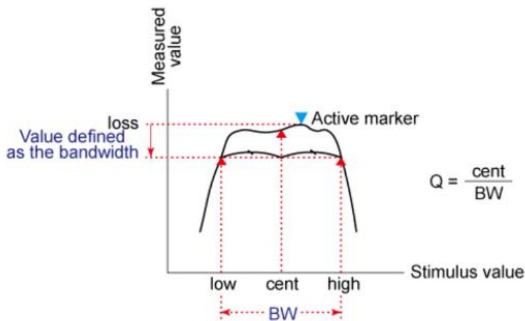
图 10-2 带宽的选择
