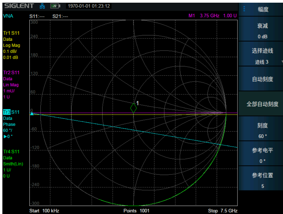
图 10-1 迹线展示
