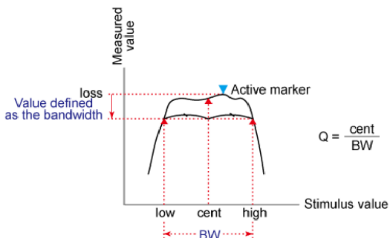
图 3-3 带宽的选择
