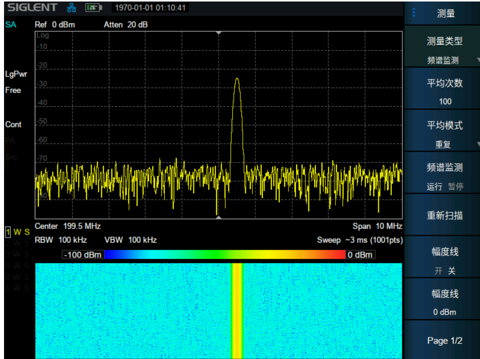
图 3-12 频谱监测
