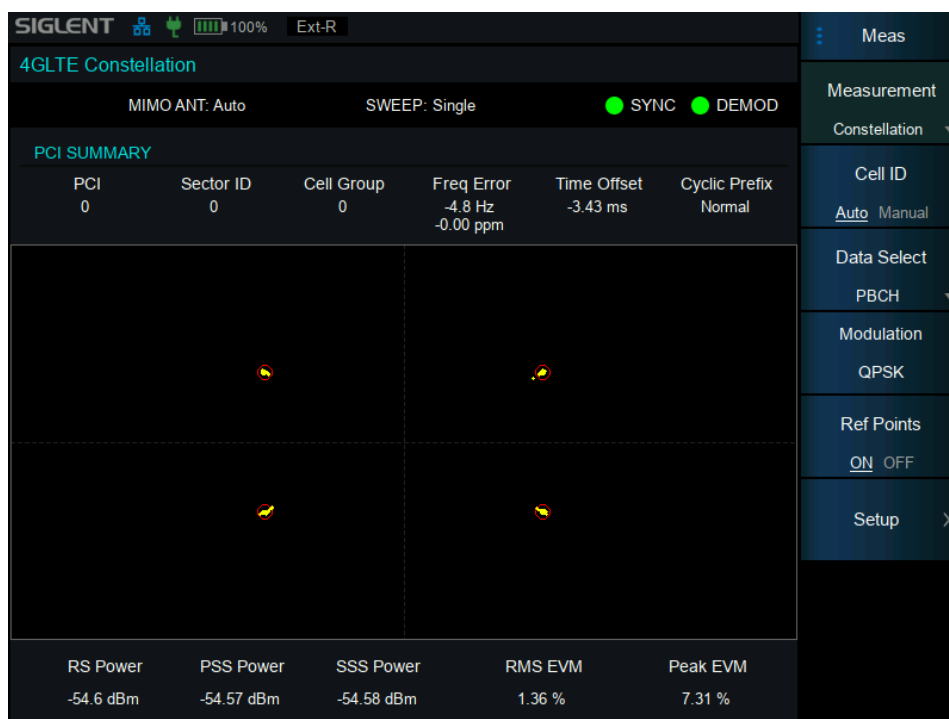
图 6-7 星座图视图
