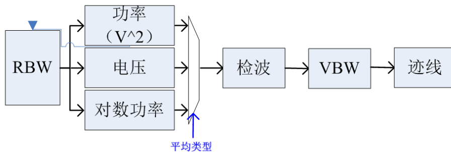
图 3-6 平均类型
