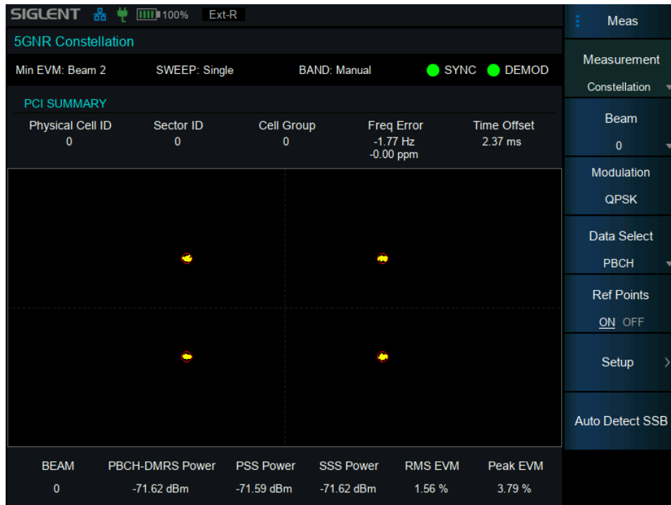
图 5-8 星座图视图
