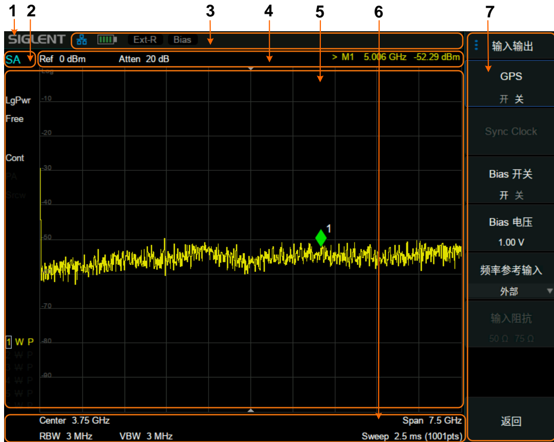
图 1-8 屏幕显示区
