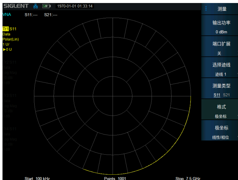
图 10-5 极坐标图
