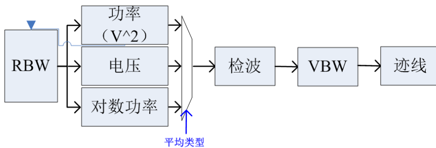
图 7-3 平均类型
