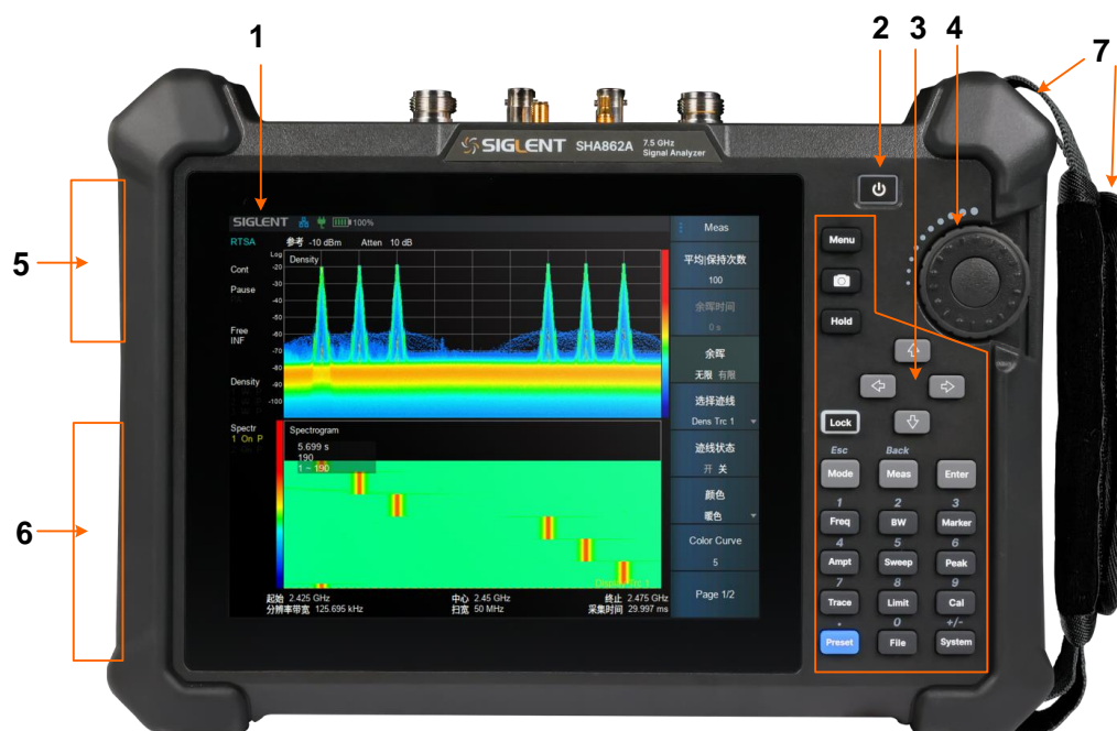
图 1-4 前面板
