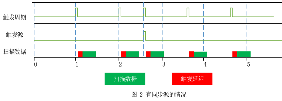
图 7-1 同步源的触发
