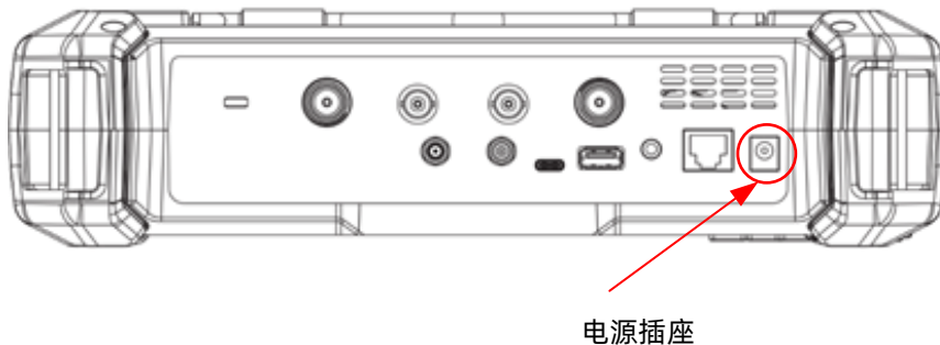
图 1-3 后视图和电源
