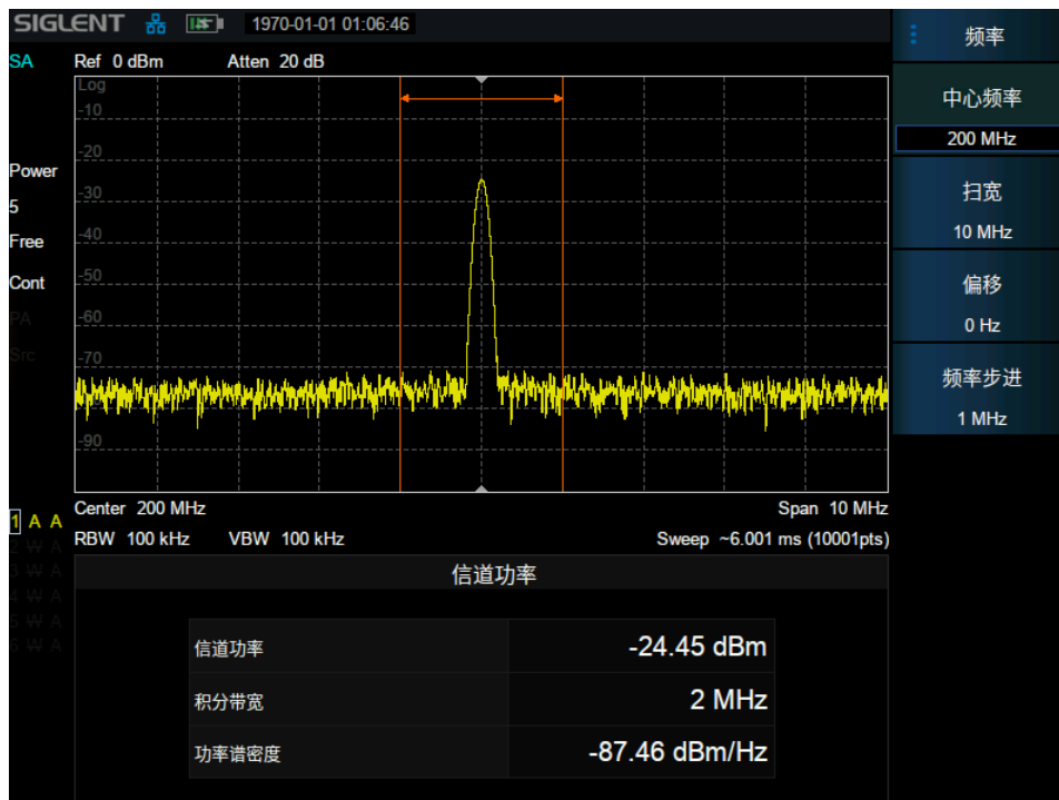
图 3-7 信道功率
