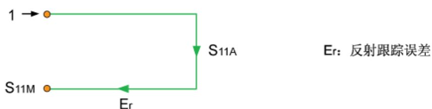
图 10-6 开路校准
