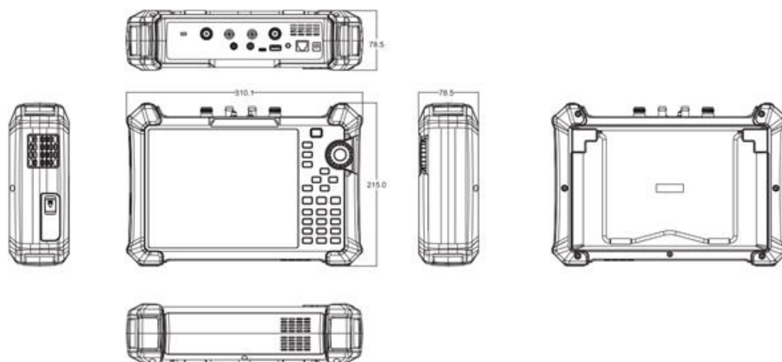
图 1-1 正侧视图
