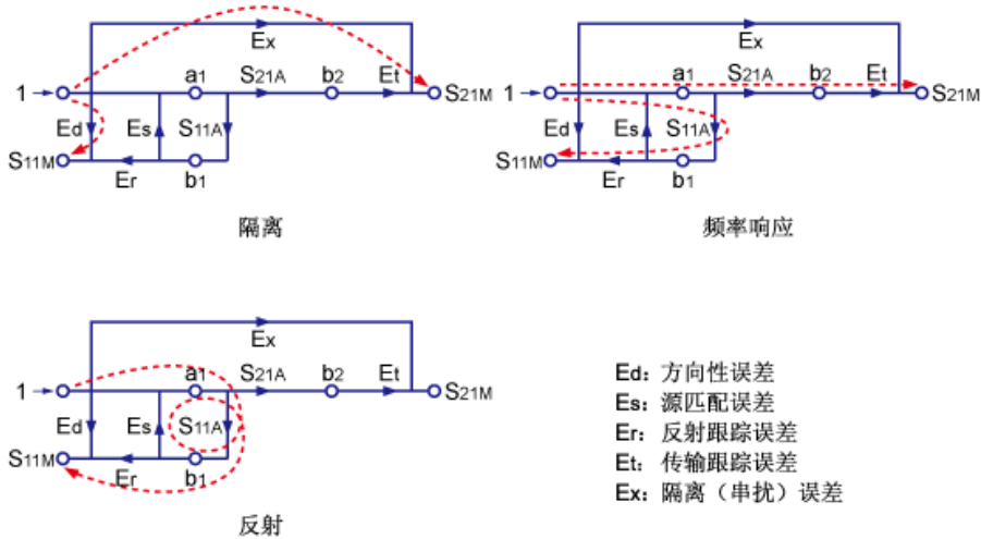
图 9-6 增强校准模型
