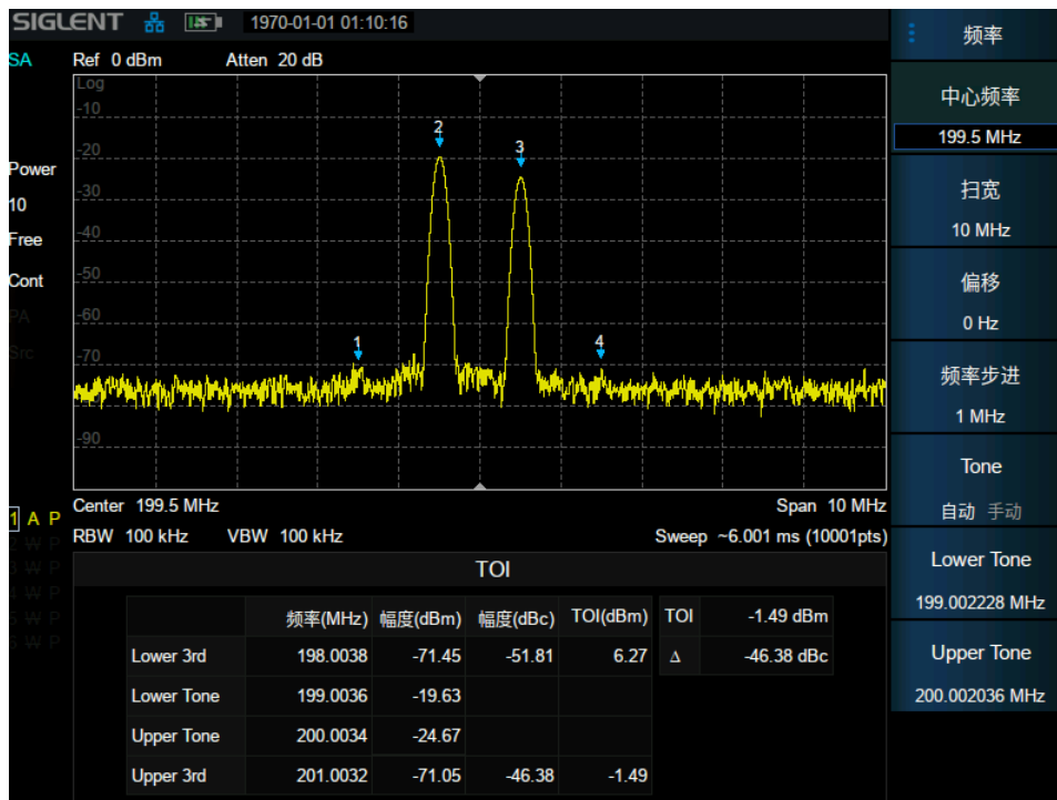
图 3-11 三阶交调
