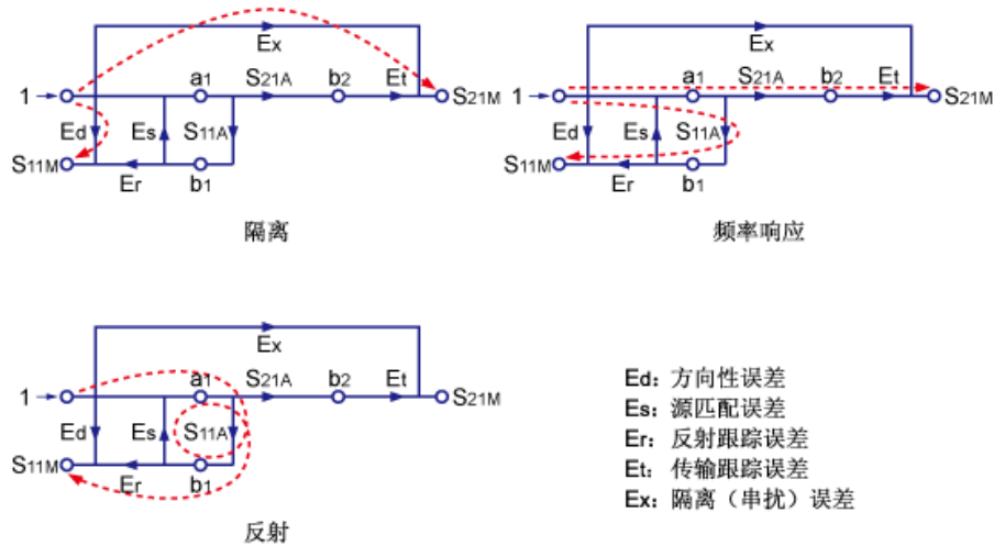
图 10-10 增强校准模型
