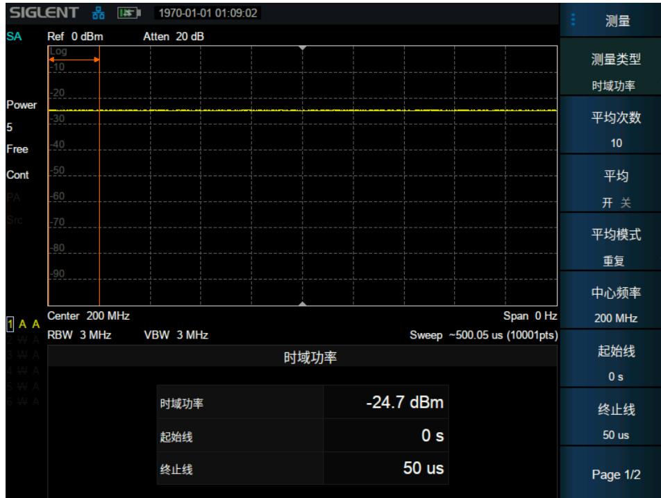
图 3-10 时域功率
