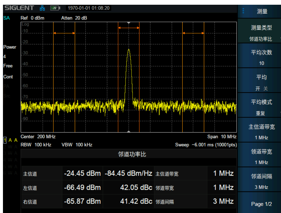
图 3-8 邻道功率比
