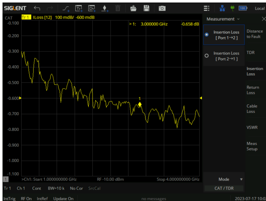
图 11-6 插入损耗测量界面
