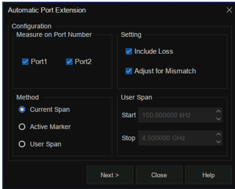
图 6-30 自动端口延伸设置界面
