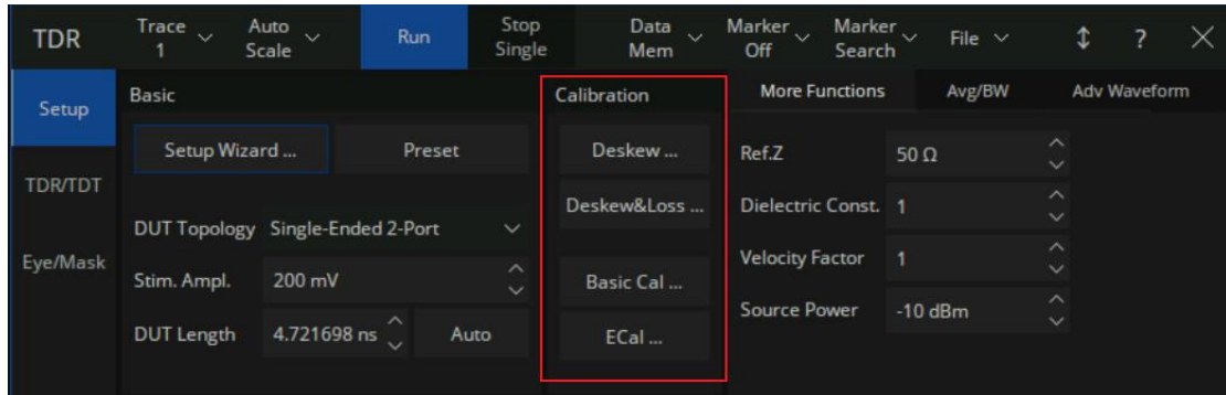
图 8-3 TDR 校准按钮
