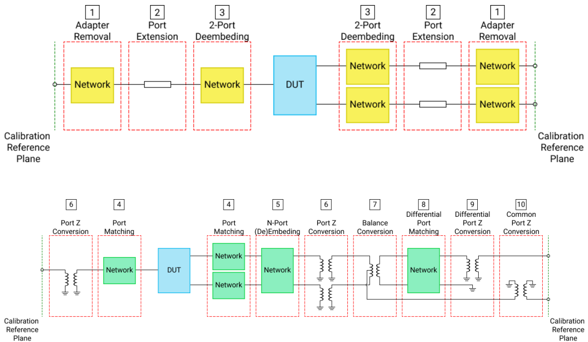
图 6-1 功能应用顺序示意图
