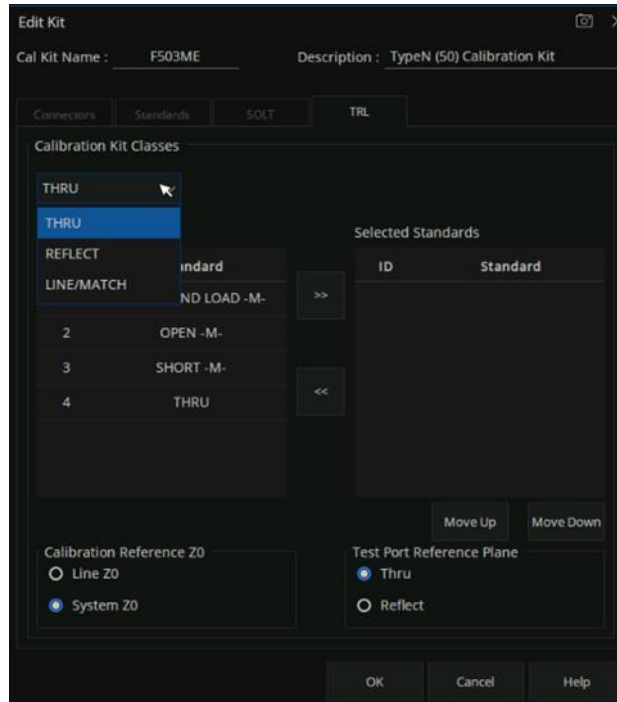
图 6-12 TRL 选项卡对话框界面
