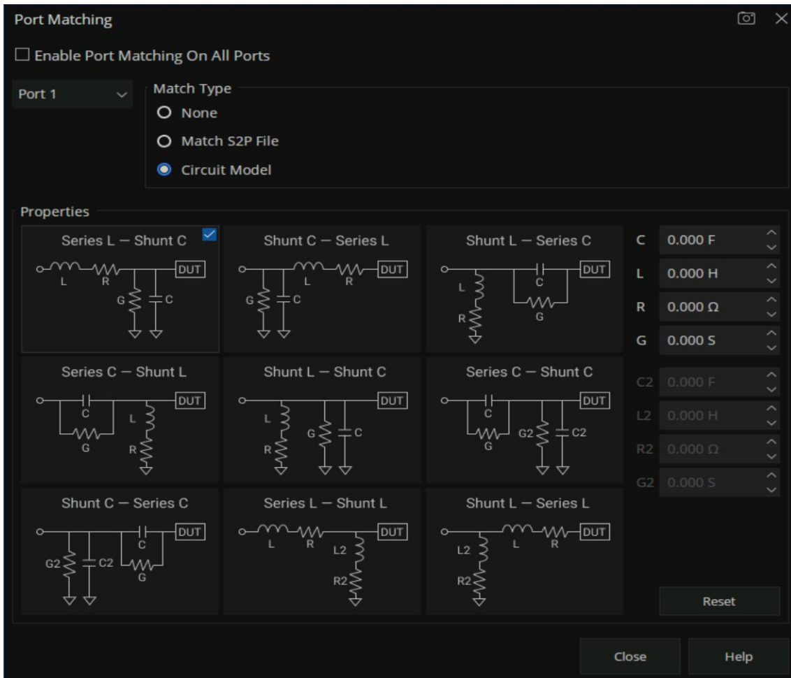
图 6-32 端口匹配
