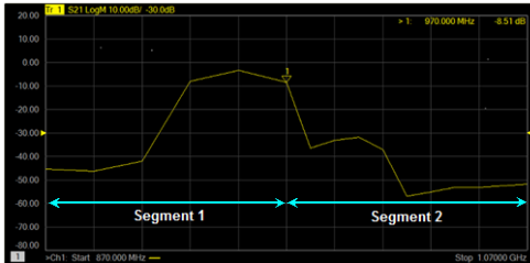
图 5-2 不使用 X 轴点间距
