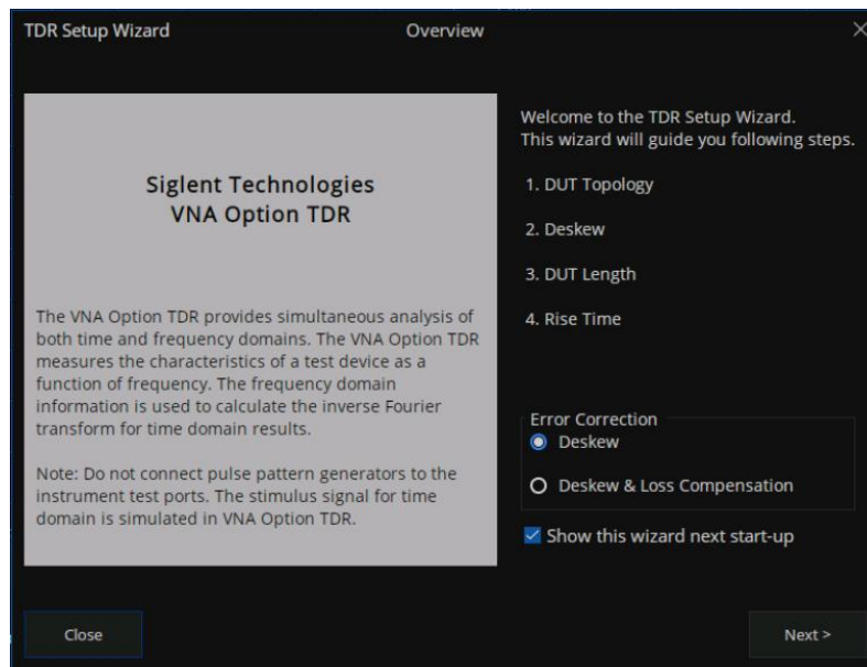
图 8-2 TDR 配置向导
