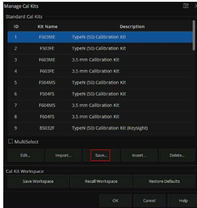
图 6-13 自定义校准件对话框界面
