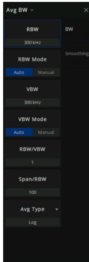
图 9-4 频谱分析信号处理相关参数设置
