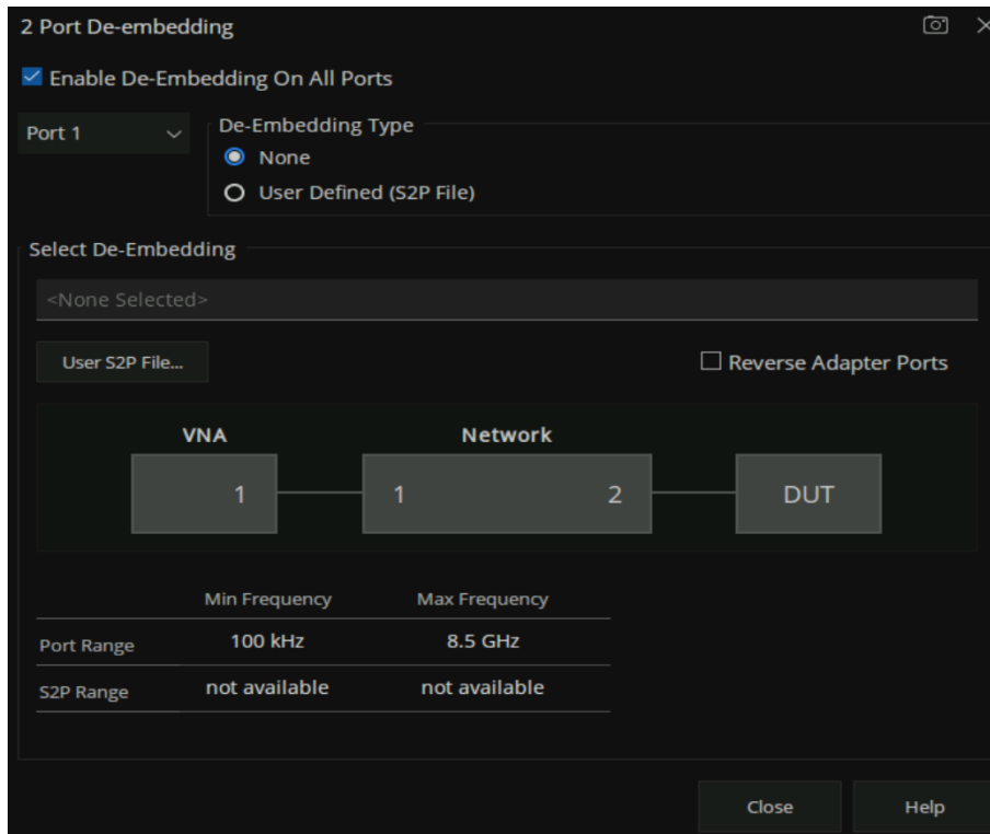
图 6-34 去嵌入界面
