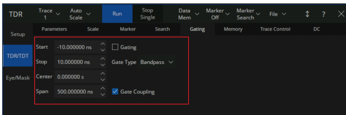
图 8-12 时域门控设置
