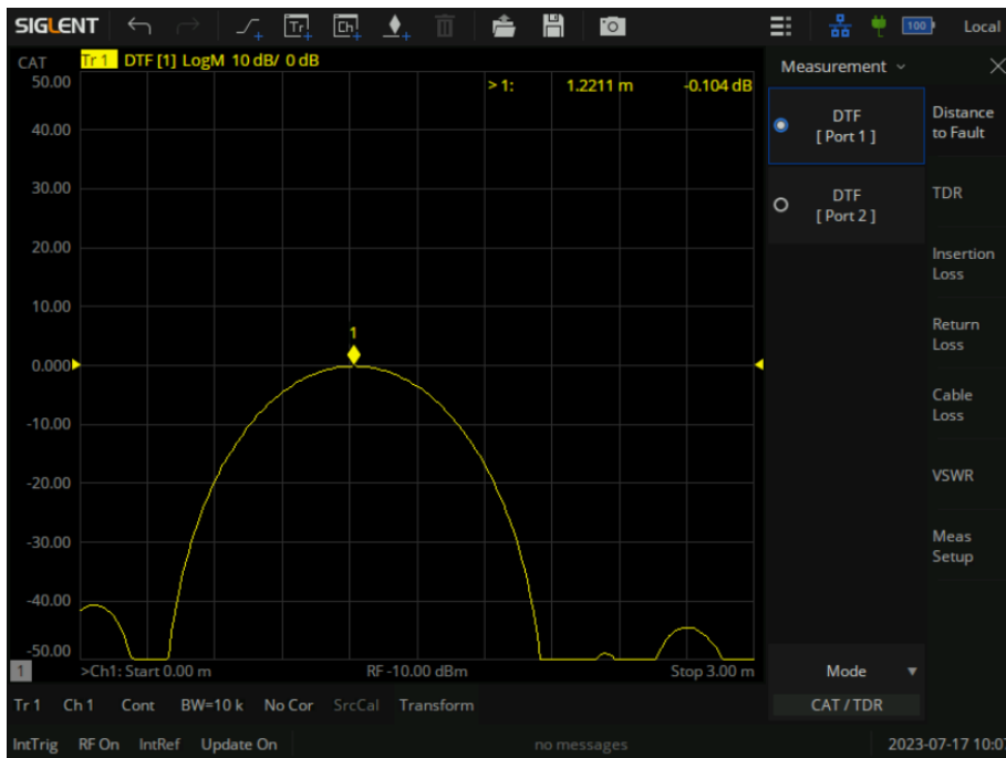
图 11-2 故障点距离测量界面
