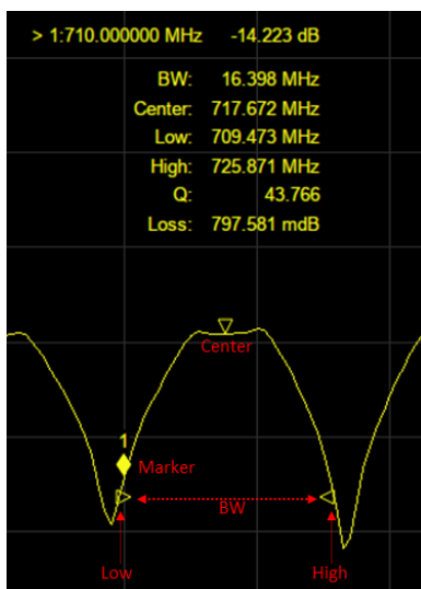
图 7-2 带宽搜索示例
