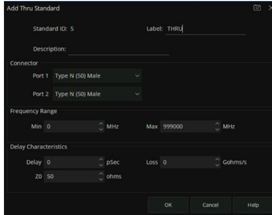
图 6-9 THRU 特性界面
