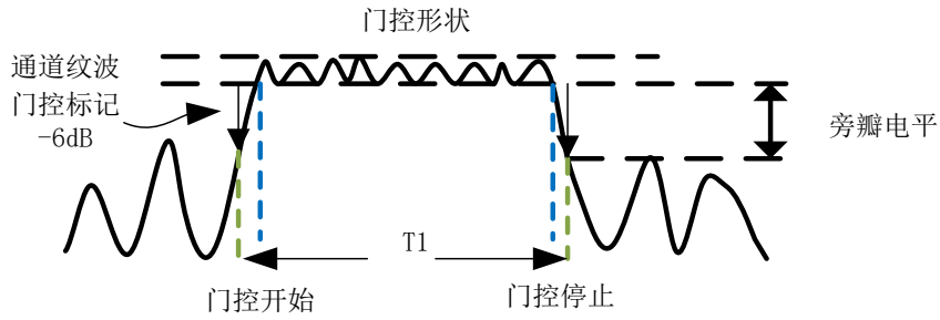
图 7-15 门控示意图
