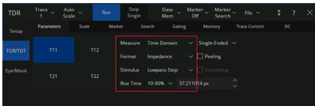
图 8-10 TDR 迹线测量设置
