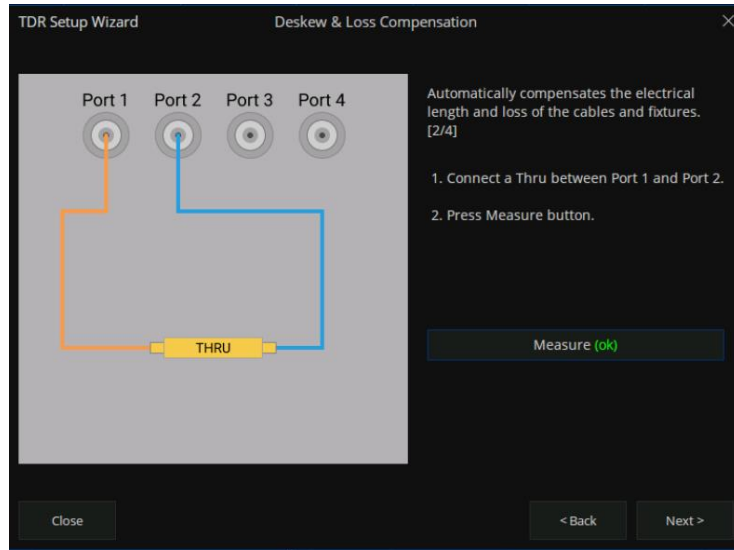
图 8-5 TDR 延时损耗补偿校准向导
