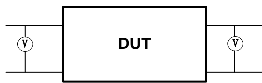
Fig2.2 平衡设备
