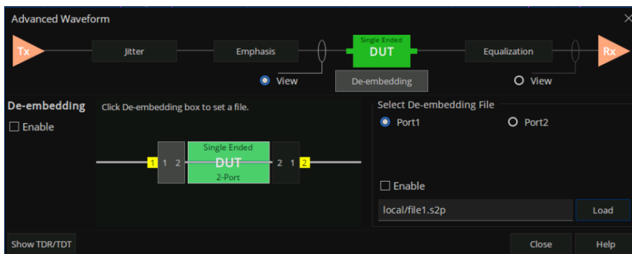
图 8-17 TDR 去嵌入设置
