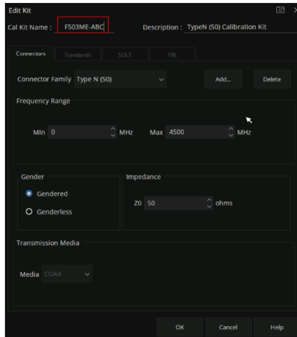
图 6-16 编辑新导入校准件示意图
