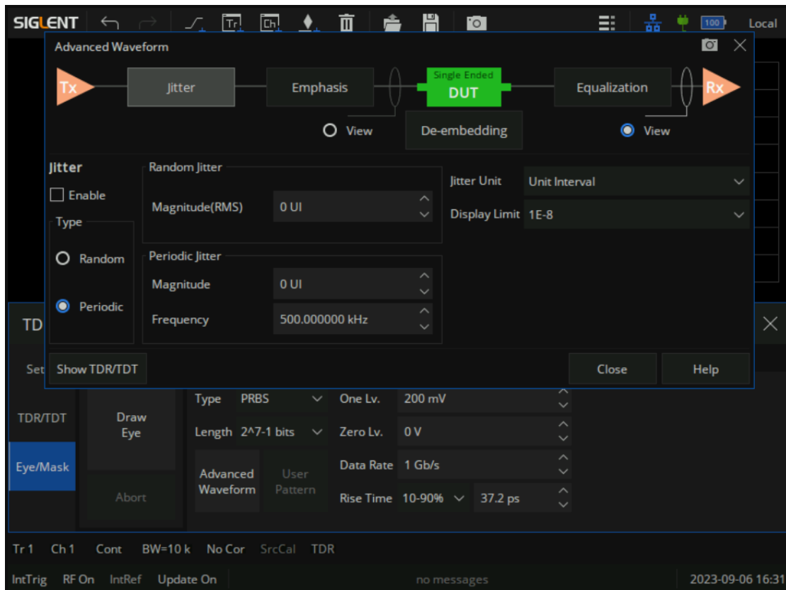
图 8-15 眼图抖动设置
