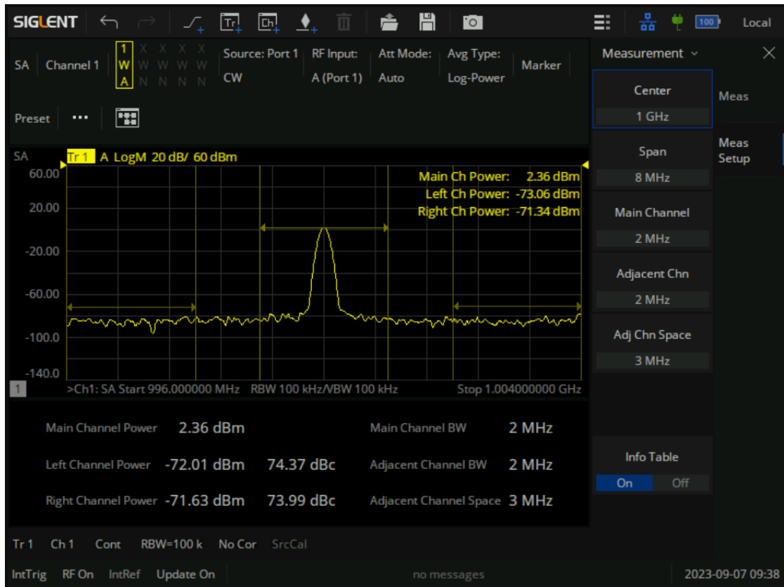
图 9-13 ACPR 测量界面
