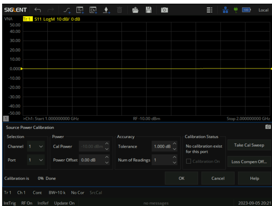
图 6-26 发射机功率校准
