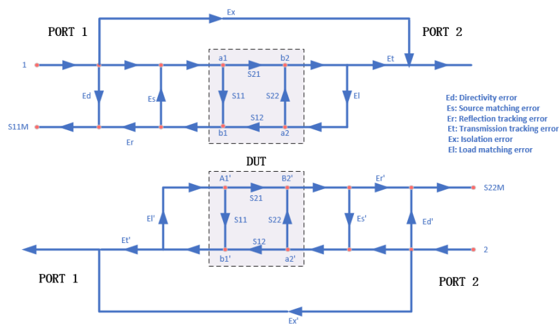
图 6-25 误差模型示意图
