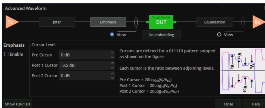
图 8-16 TDR 去加重/预加重设置
