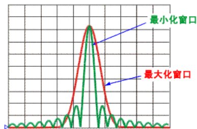
图 7-17 最大最小窗口示意图
