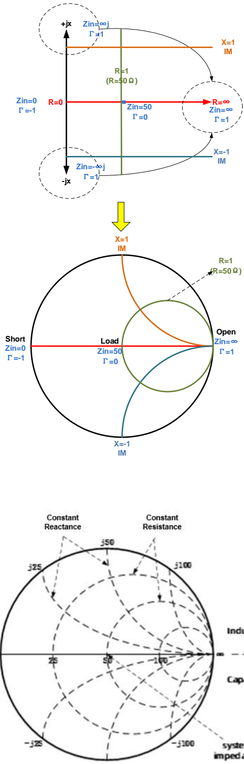
图 5-5 史密斯圆图示意图
