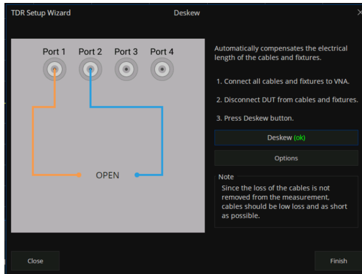
图 8-4 TDR 延时补偿校准向导
