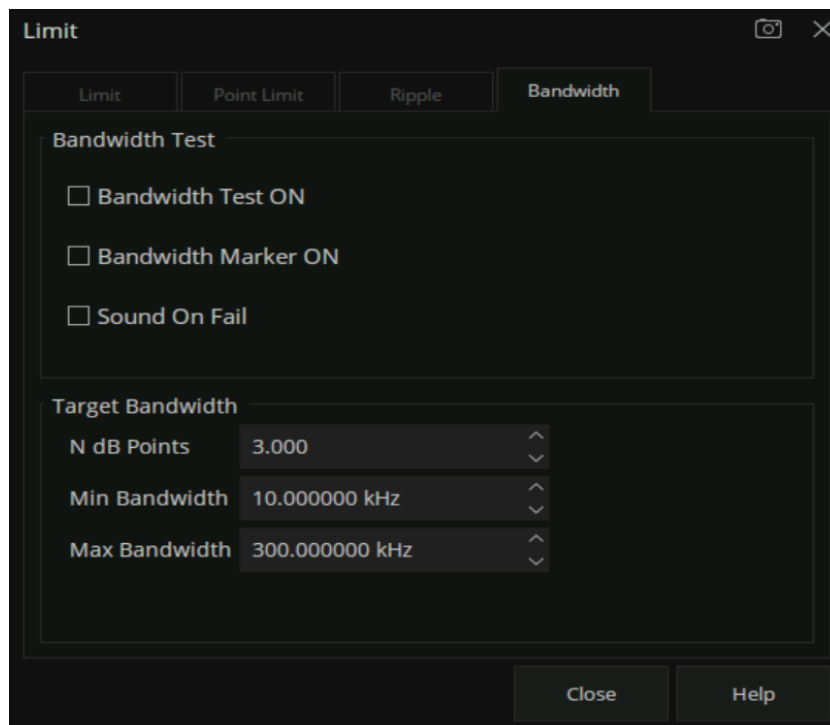
图 7-12 带宽测试设置界面
