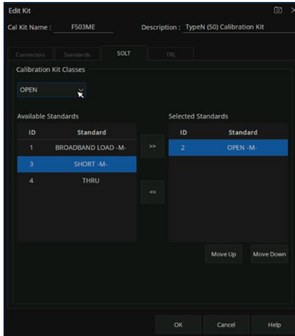
图 6-11 SOLT 选项卡对话框界面
