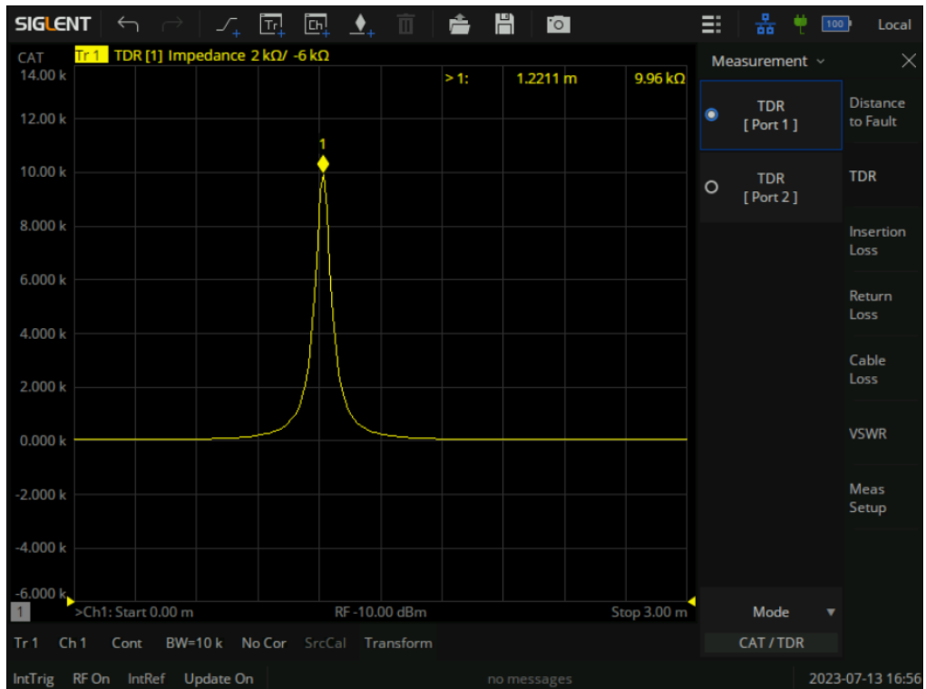
图 11-4 时域反射计测量界面
