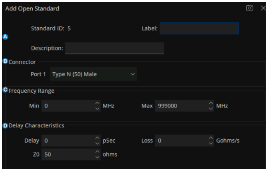
图 6-5 标样帮助对话框界面
