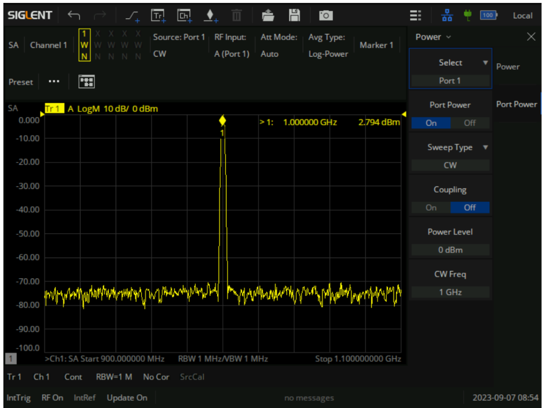
图 9-8 通过按【Power】键进入端口功率设置菜单
