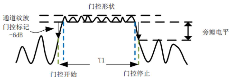
图 11-5 门控参数定义
