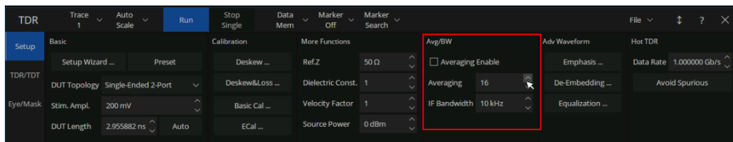
图 8-8 平均与中频带宽
