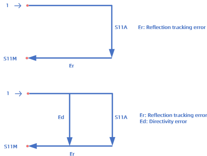
图 6-22 示意图
