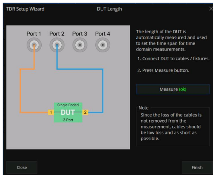
图 8-7 DUT 长度测量向导
