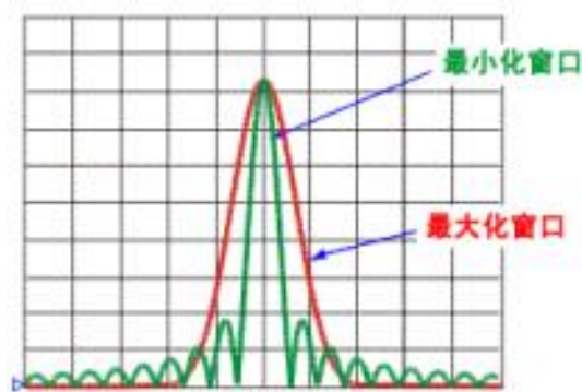
图 11-3 凯瑟窗
