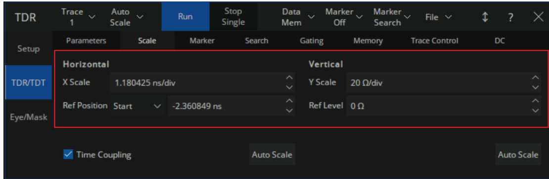
图 8-9 手动刻度设置
