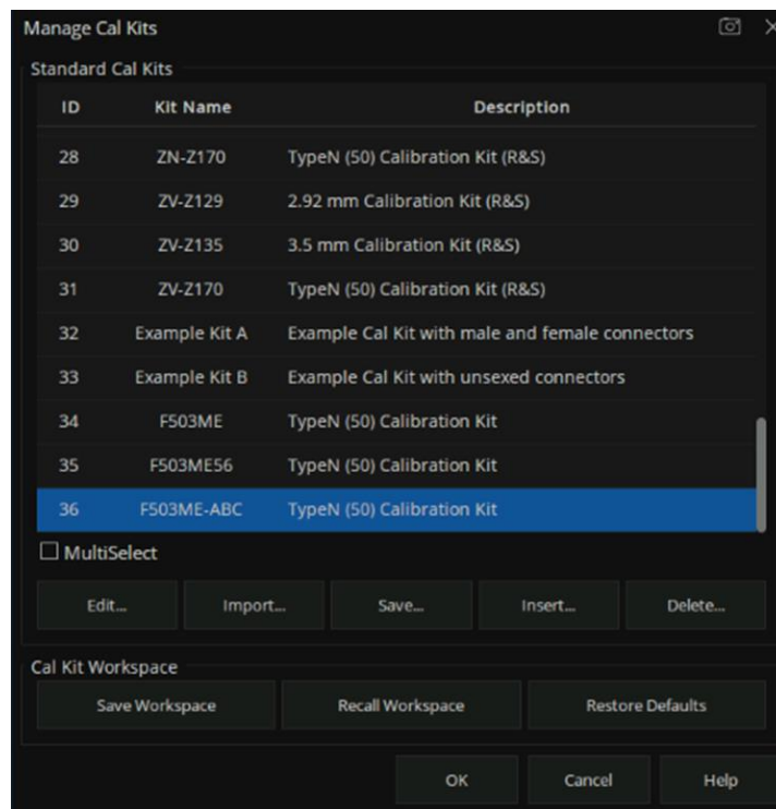
图 6-17 查看新创建成功的校准件
