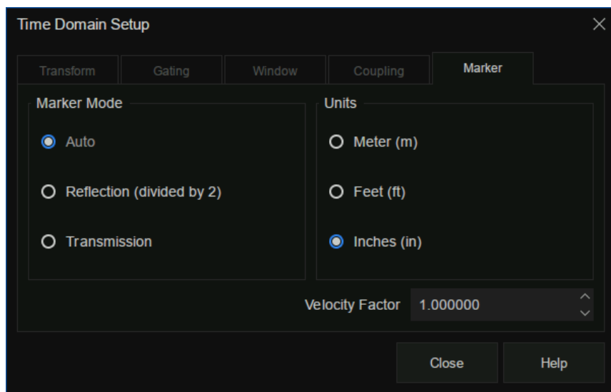
图 7-19 标记设置界面
