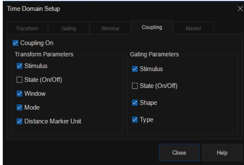
图 7-18 耦合设置界面
