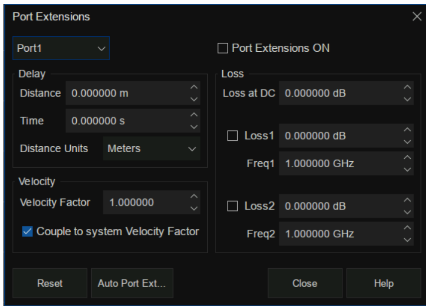
图 6-29 端口延伸设置界面
