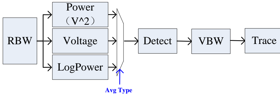
图 9-5 平均类型流程图
