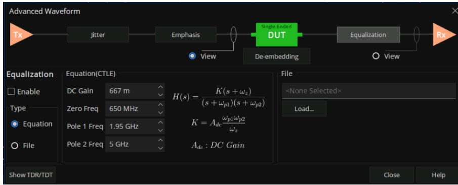
图 8-18 TDR 均衡设置
