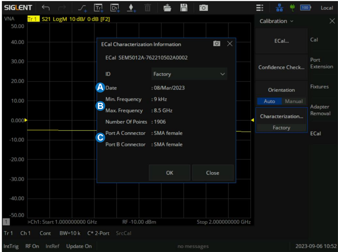
图 6-43 查看 ECal 出厂参数
