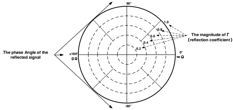
图 5-4 极坐标示意图
