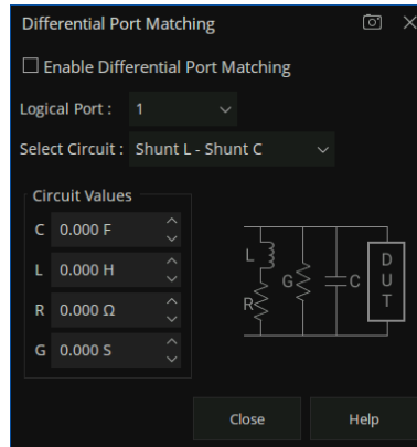
图 6-36 差模端口匹配
