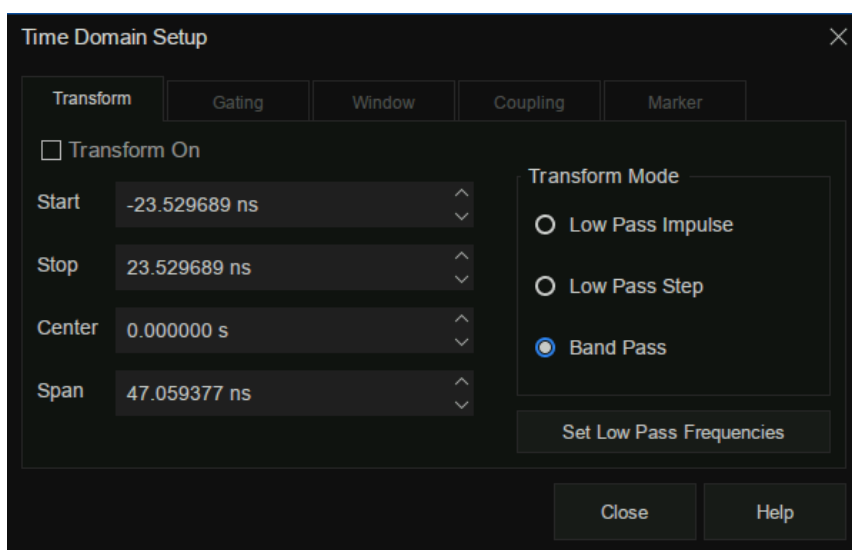
图 7-13 时域设置界面
