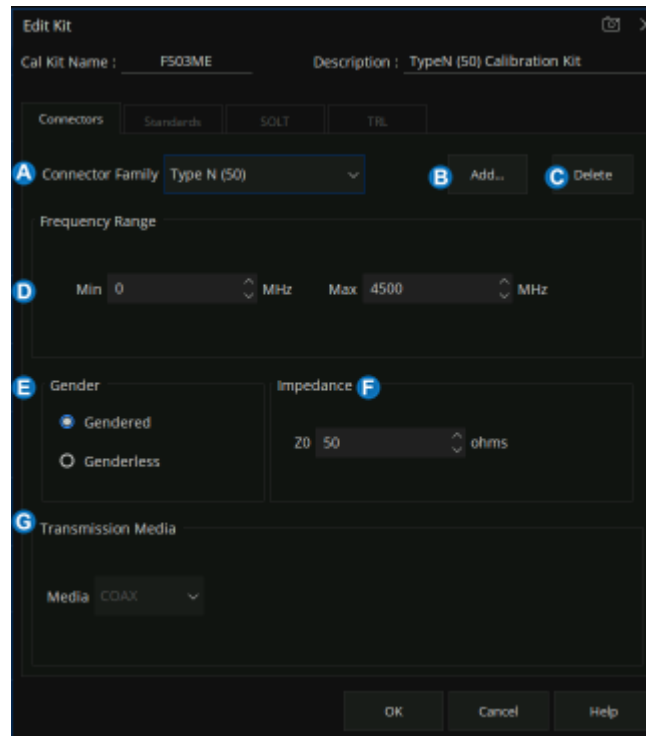
图 6-3 Connectors 选项卡界面
