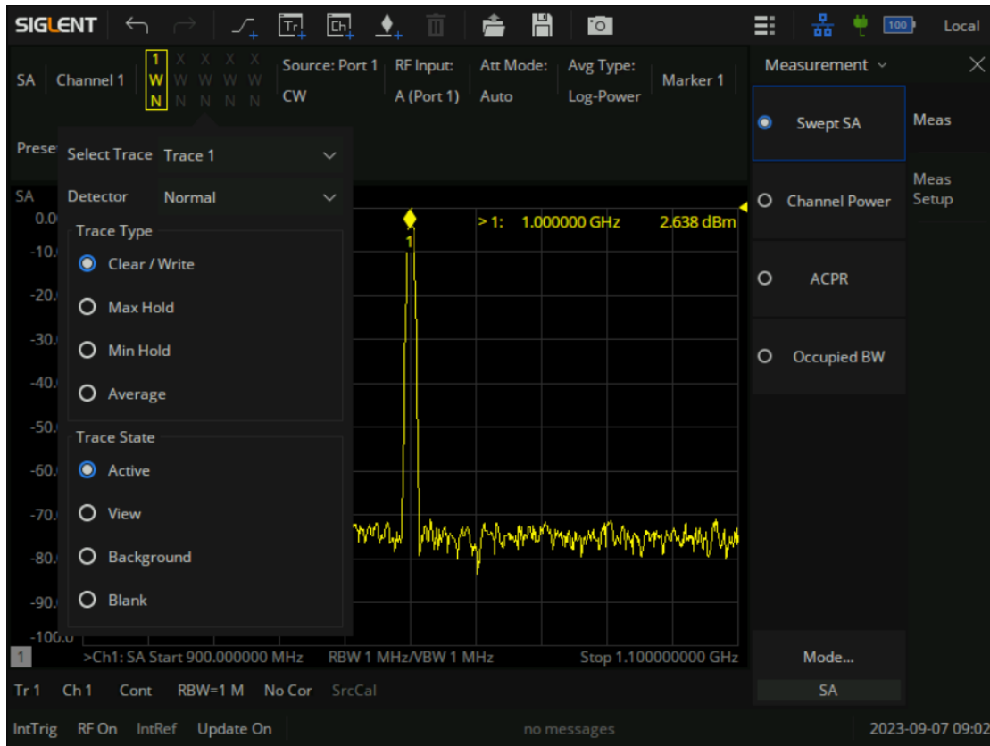
图 9-10 迹线设置下拉菜单
