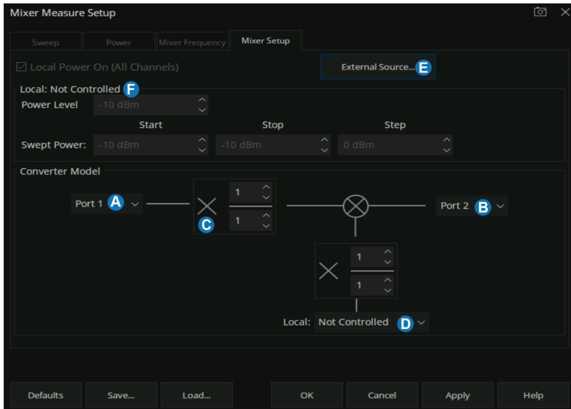
图 12-7 Mixer Setup 选项卡
