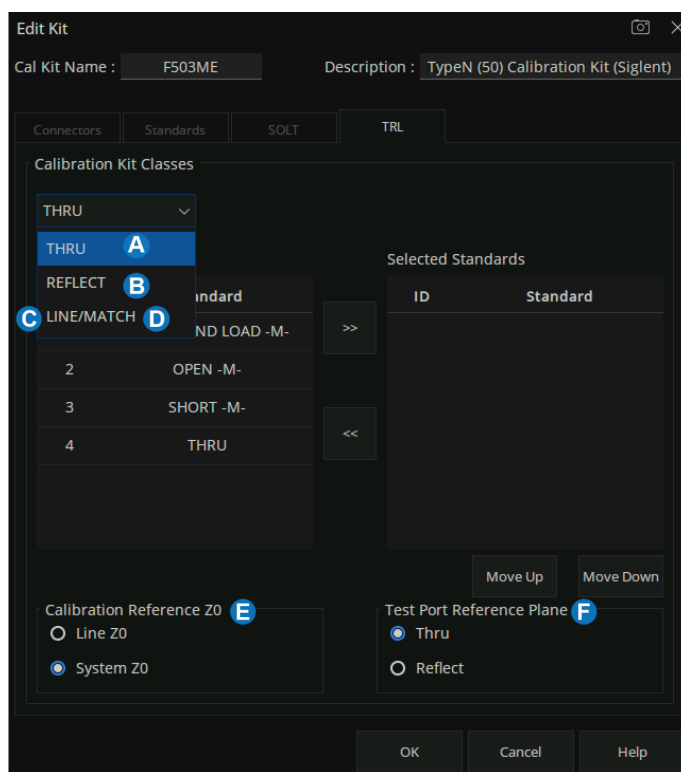
图 7-11 TRL 选项卡对话框界面
