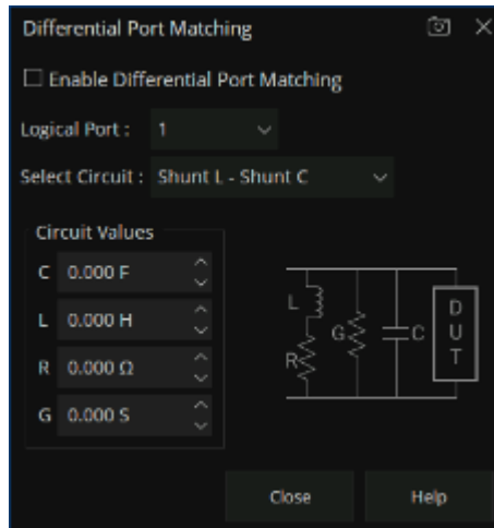
图 7-35 差模端口匹配
