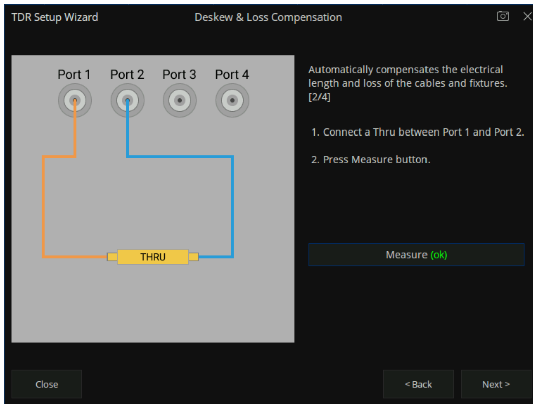
图 9-5 TDR 延时损耗补偿校准向导
