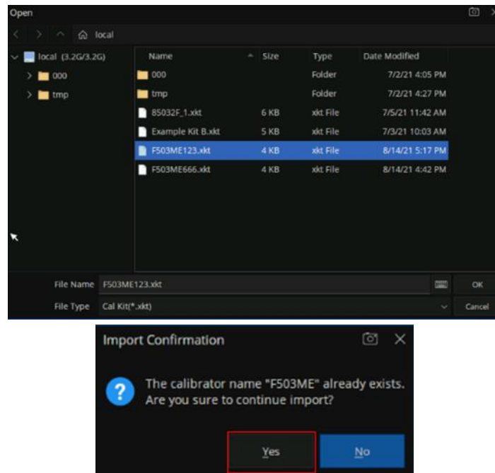
图 7-14 导入新校准件示意图
