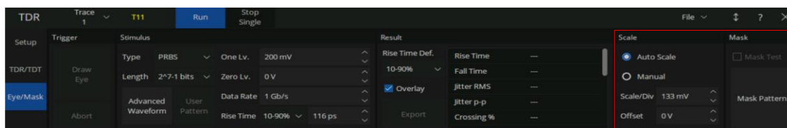
图 9-14 眼图刻度及模板设置
