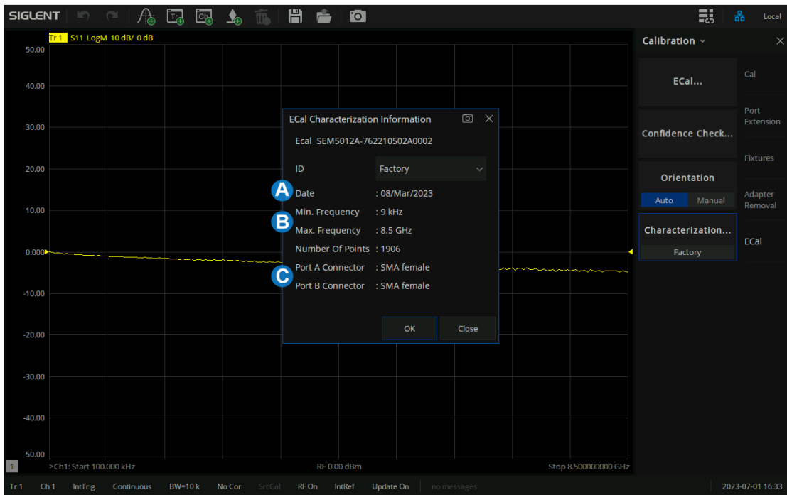
图 7-42 查看 ECal 出厂参数
