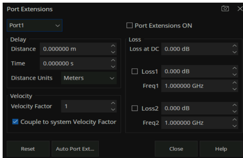
图 7-28 端口延伸设置界面
