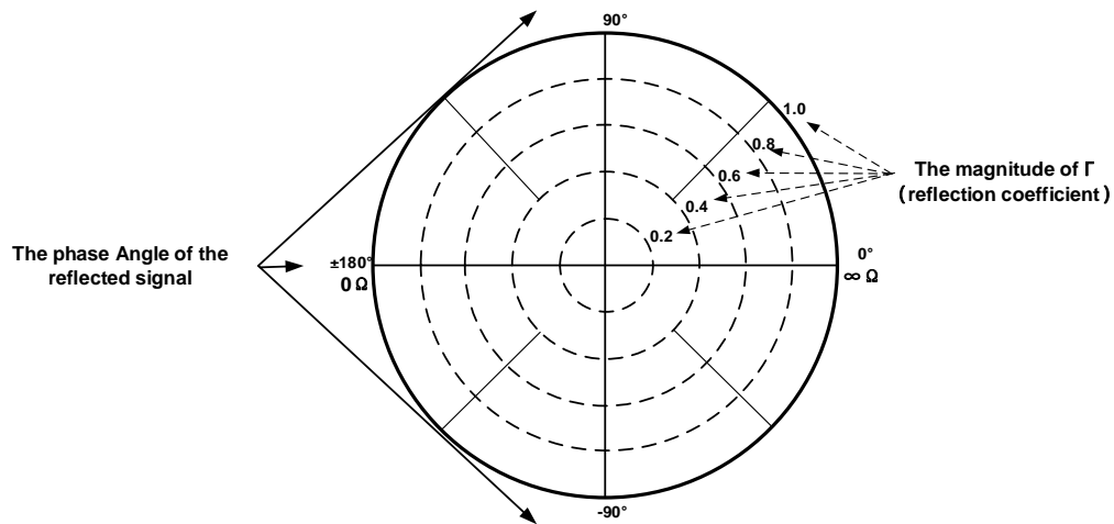
图 6-4 极坐标示意图
