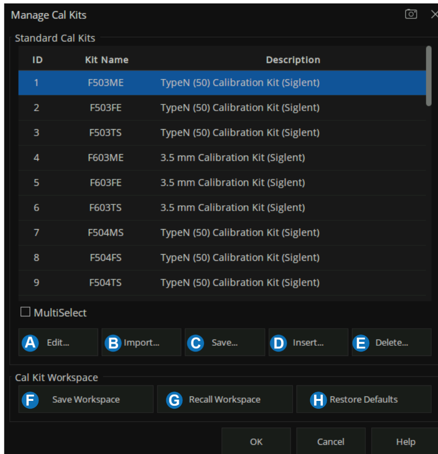
图 7-2 校准件管理界面
