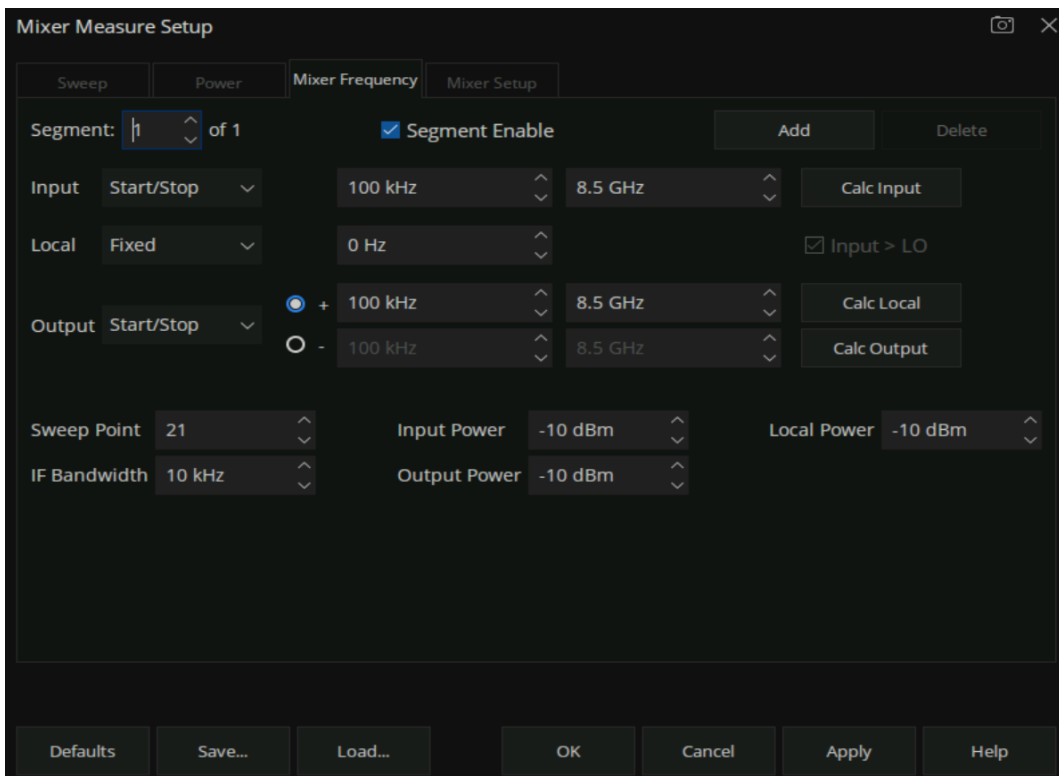
图 12-6 段扫描 Mixer Frequency 选项卡
