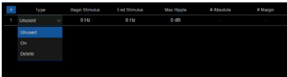
图 8-11 纹波极限线设置界面
