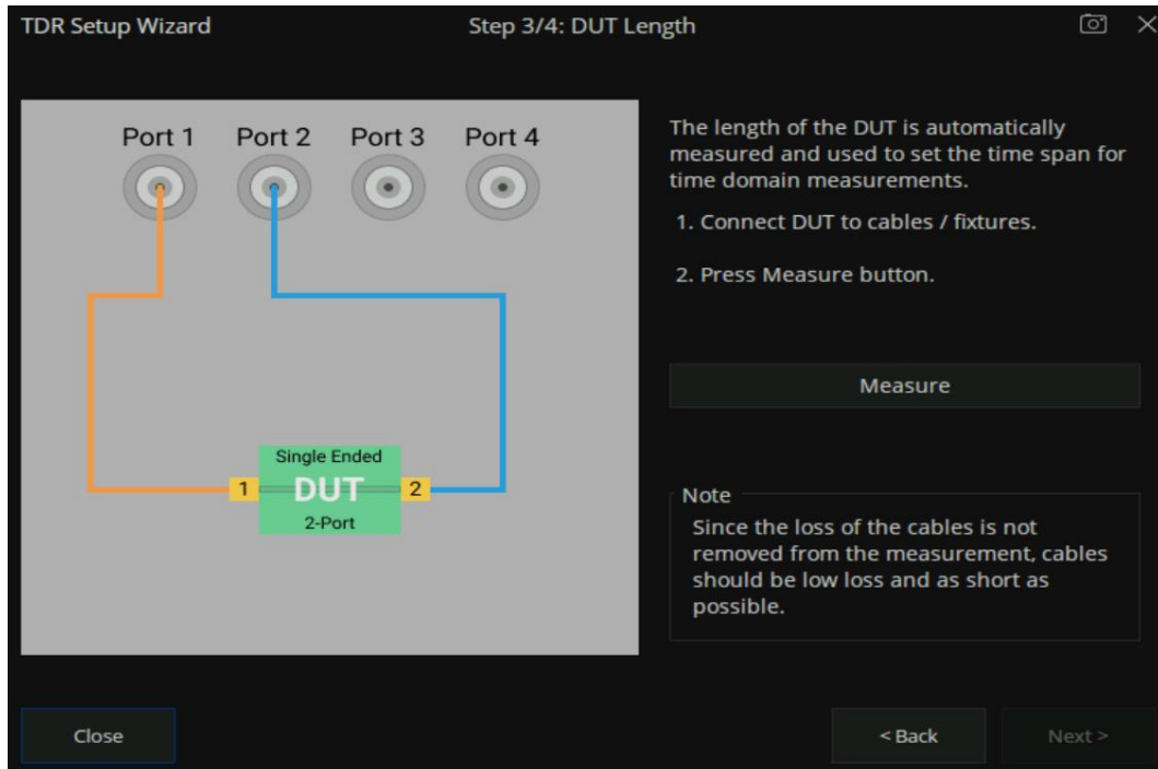
图 9-7 DUT 长度测量向导
