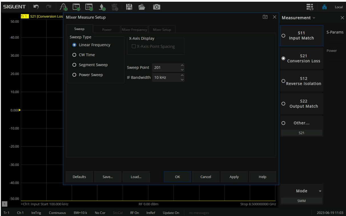
图 12-2 Mixer Measure Setup 对话框
