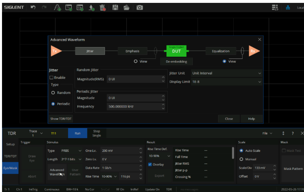
图 9-15 眼图抖动设置
