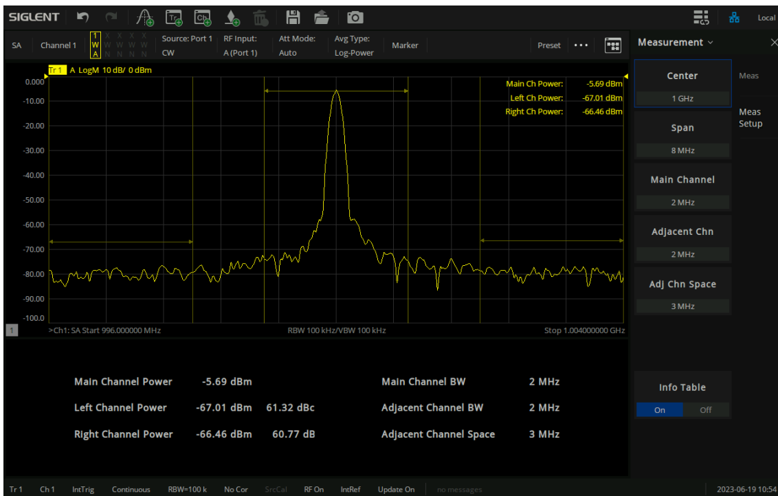
图 10-14 ACPR 测量界面
