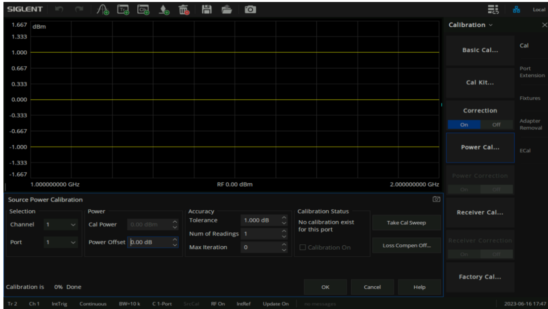
图 7-25 发射机功率校准
