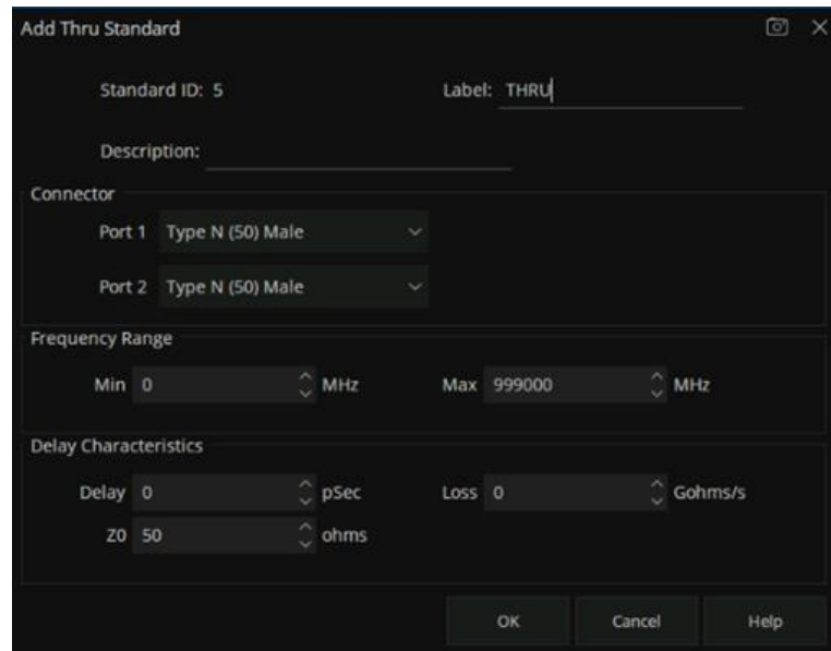
图 7-9 THRU 特性界面
