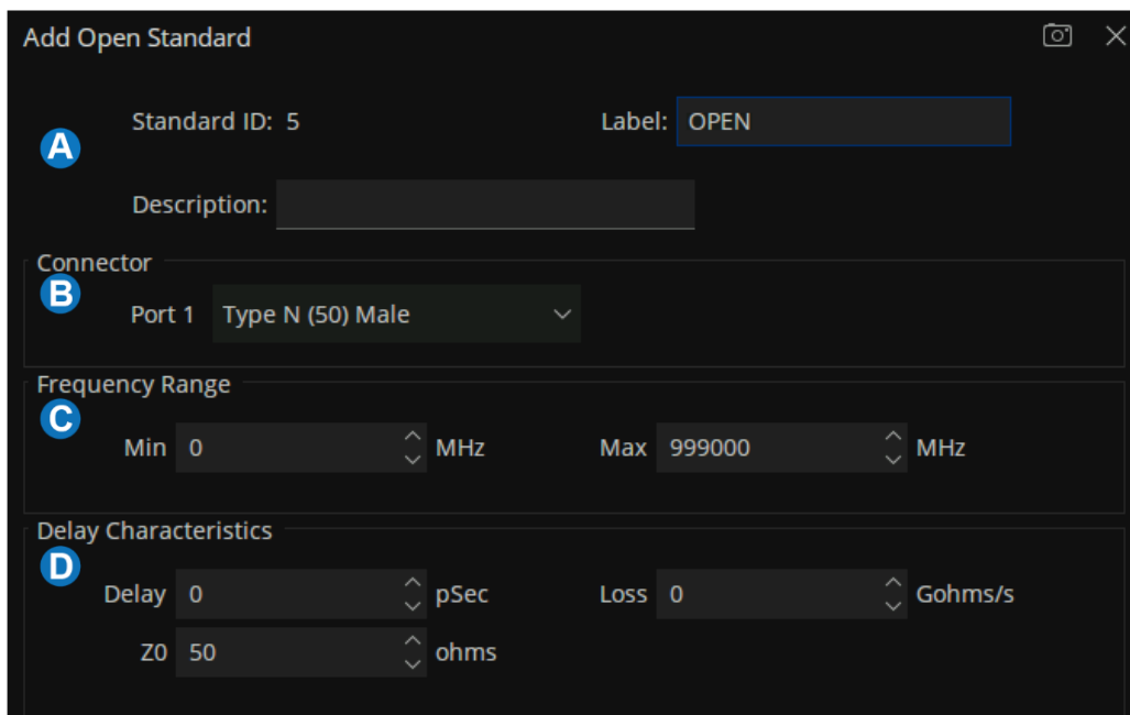
图 7-5 标样帮助对话框界面
