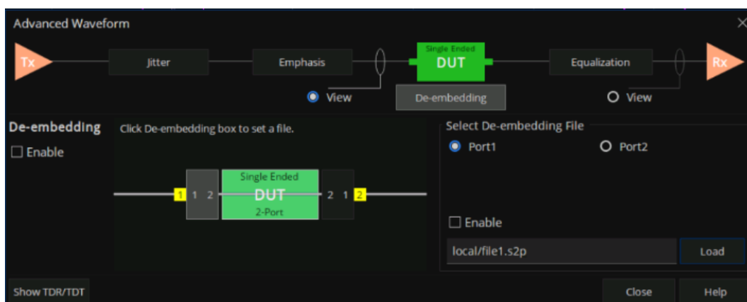
图 9-17 TDR 去嵌入设置
