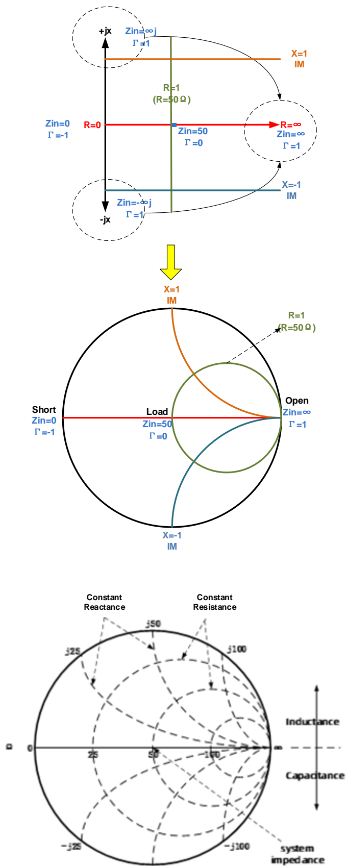
图 6-5 史密斯圆图示意图
