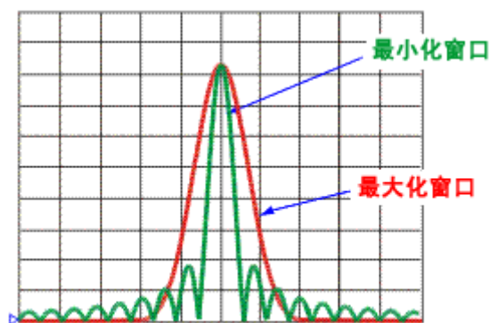
图 8-17 最大最小窗口示意图
