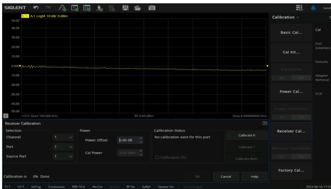
图 7-27 接收机校准设置界面
