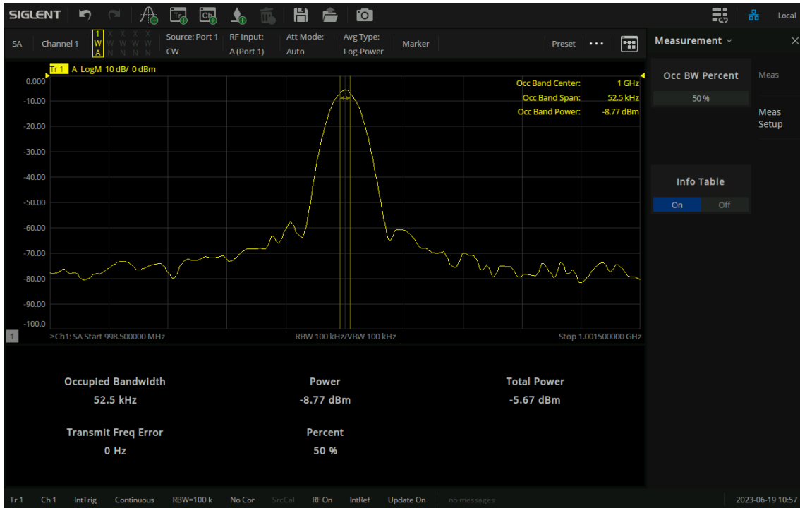
图 10-15 Occupied BW 测量界面
