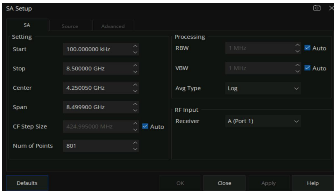
图 10-3 SA Setup 的 SA 选项卡设置界面
