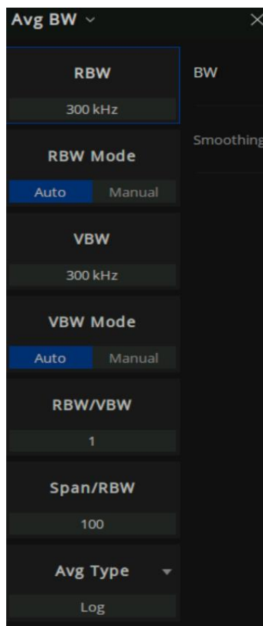
图 10-5 频谱分析信号处理相关参数设置
