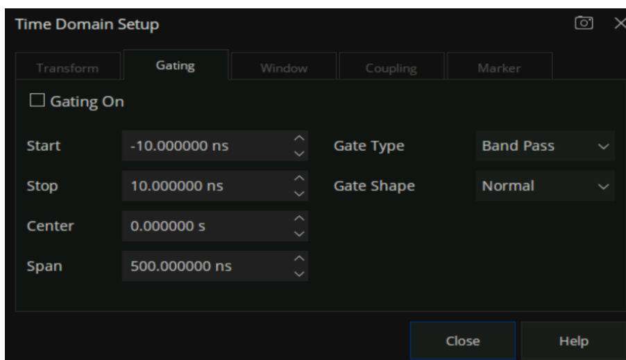
图 8-14 门控设置界面
