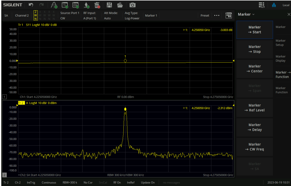
图 10-12 Marker →SA 界面
