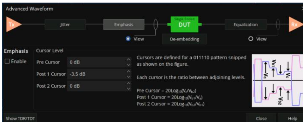
图 9-16 TDR 去加重/预加重设置
