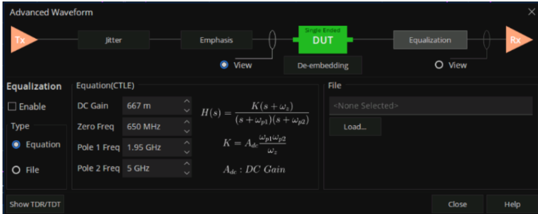
图 9-18 TDR 均衡设置
