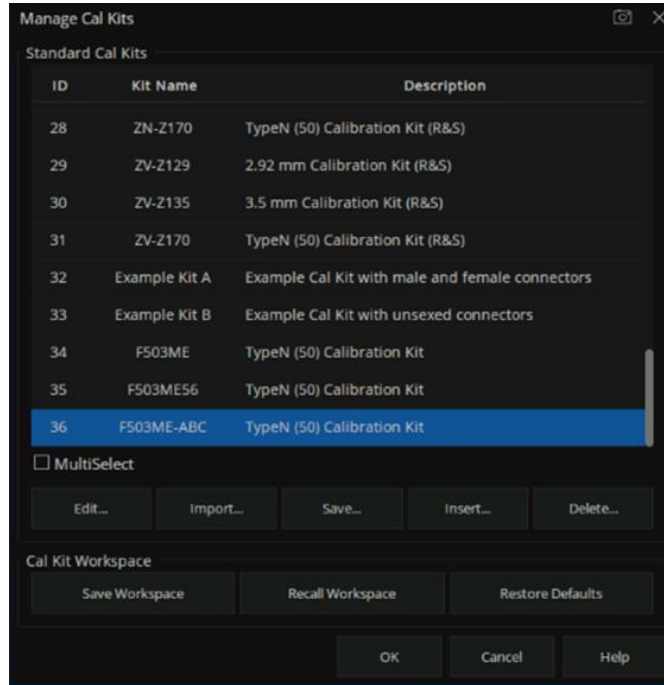
图 7-16 查看新创建成功的校准件
