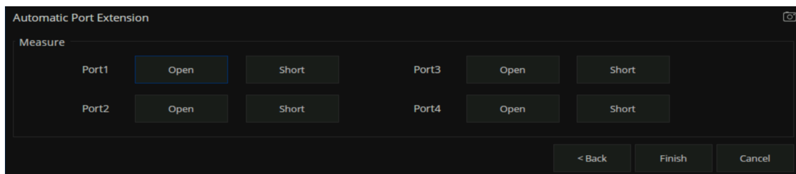
图 7-30 自动端口延伸校准界面
