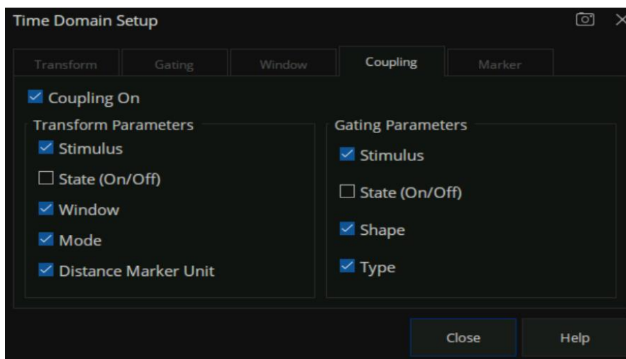
图 8-18 耦合设置界面
