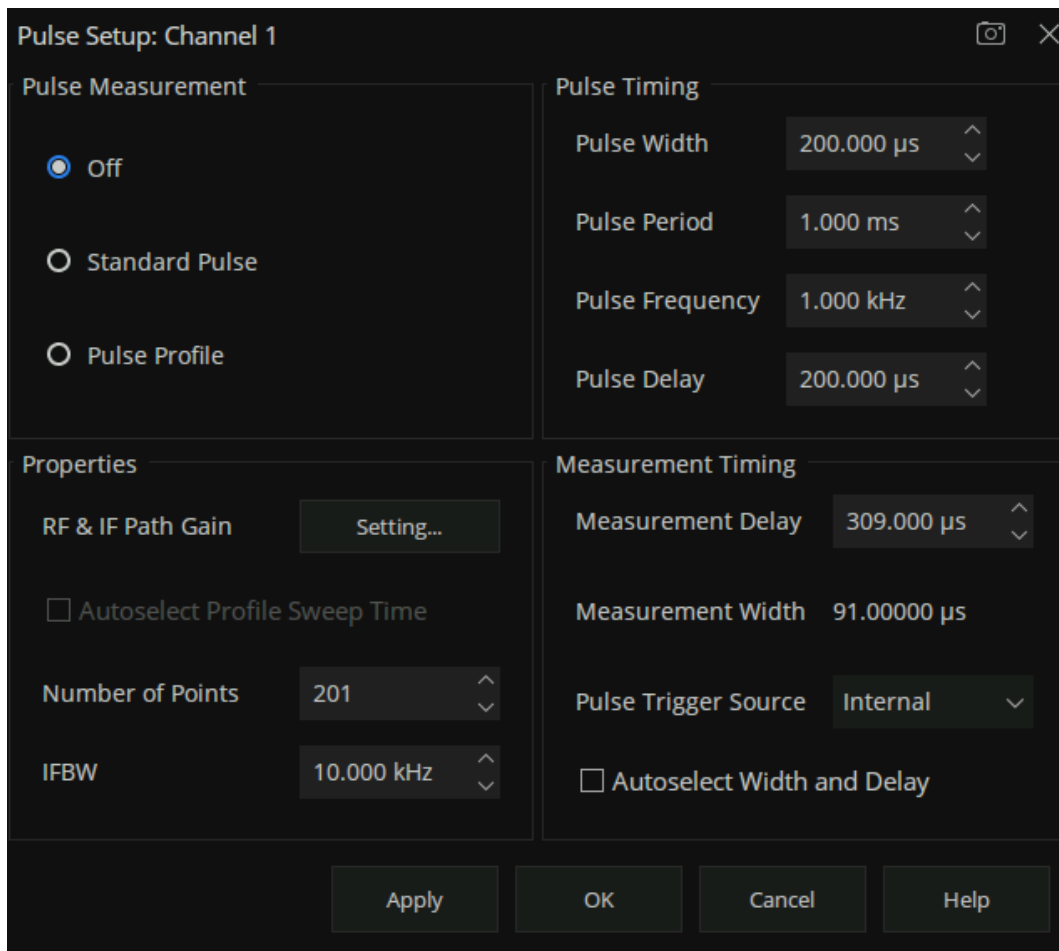
图 13-1 脉冲测量设置界面
