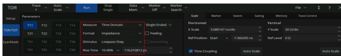
图 9-10 TDR 迹线测量设置
