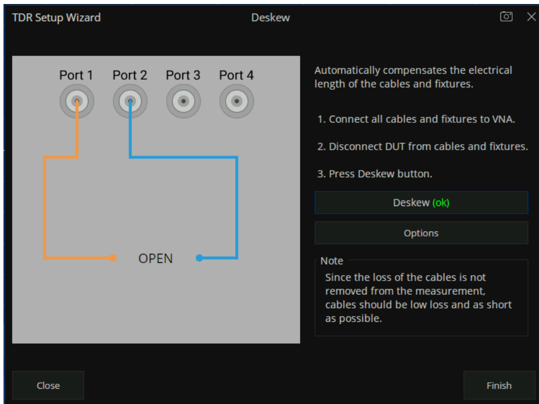
图 9-4 TDR 延时补偿校准向导
