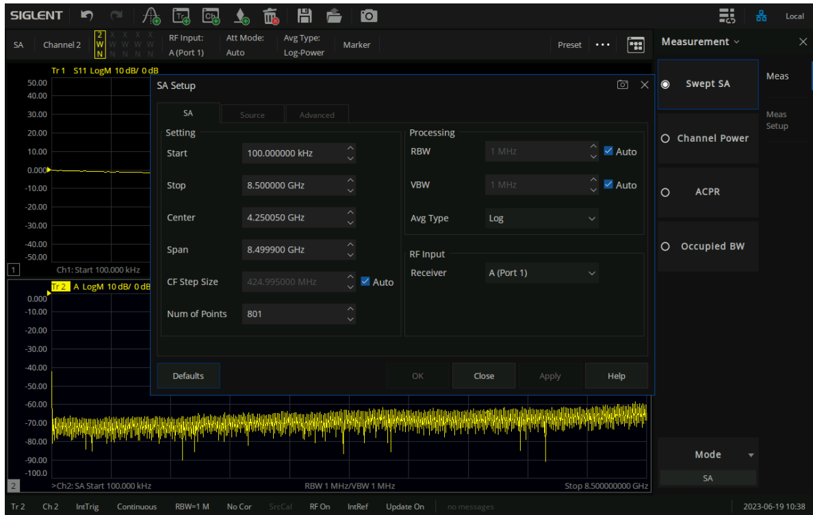
图 10-2 SA Setup 对话框
