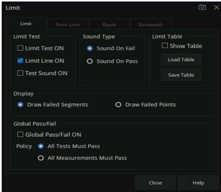
图 8-6 极限测试界面
