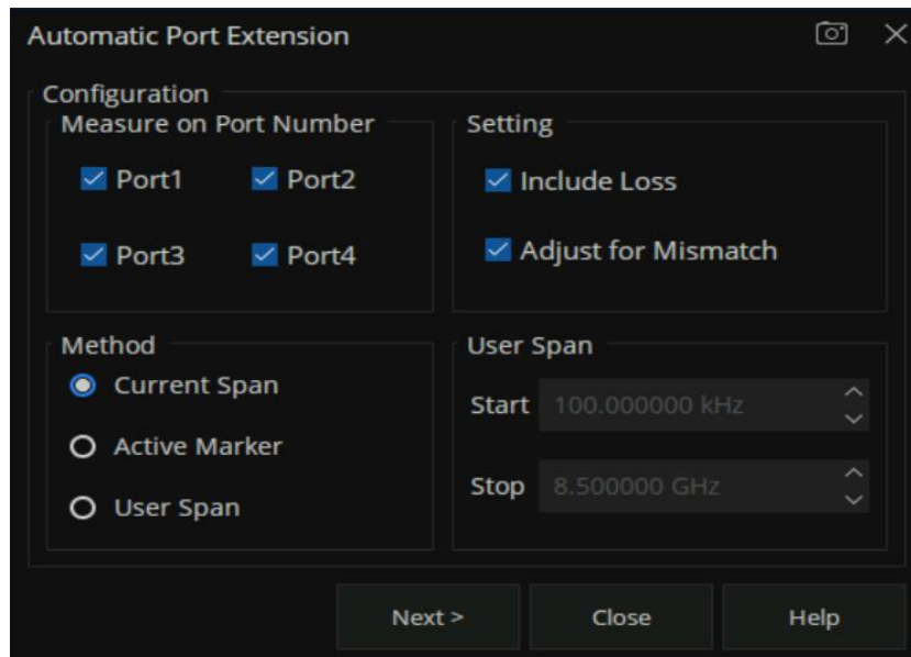
图 7-29 自动端口延伸设置界面
