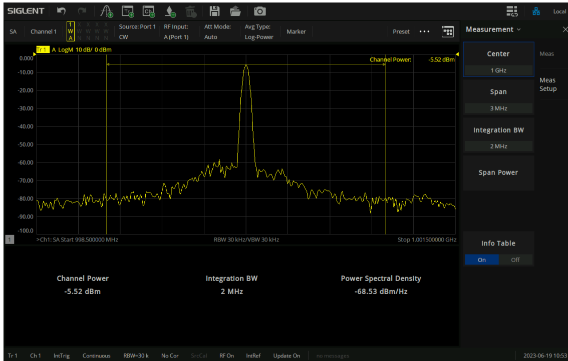
图 10-13 Channel Power 界面
