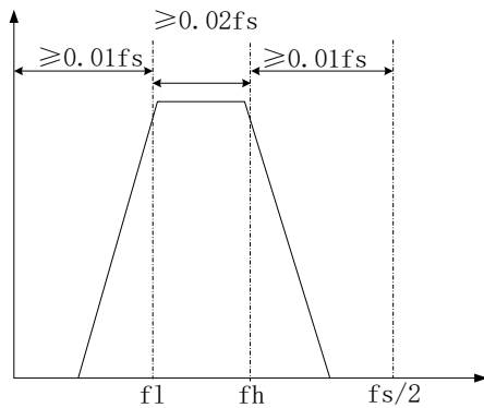
带通
