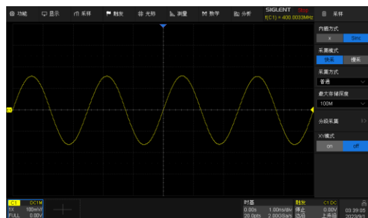
Sinc 插值
