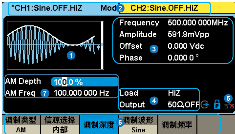
图 4 SDG6000X 触摸屏显示区
