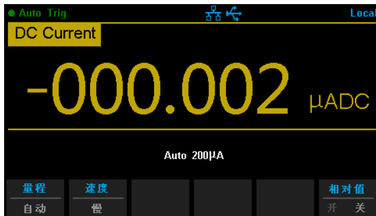
图 2-6 直流电流测量界面
