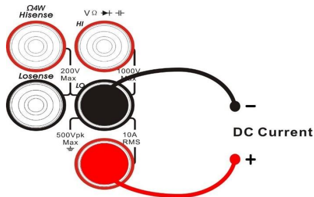
图 2-7 直流电流测量连接示意图
