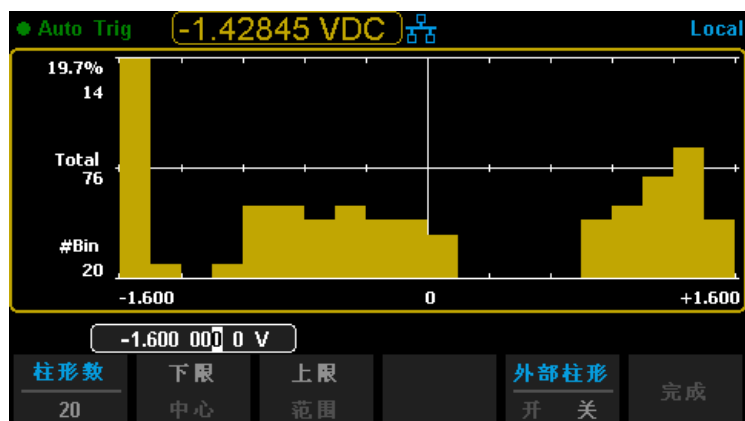
图 2-81 柱形设置界面
