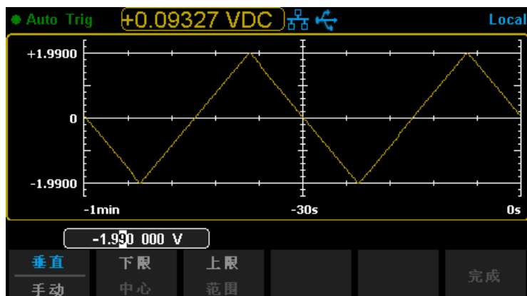
图 2-79 手动设置垂直刻度
