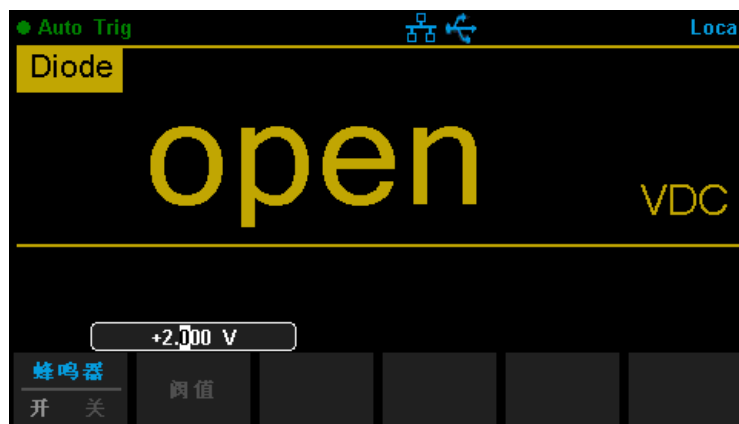
图 2-25 检查二极管界面
