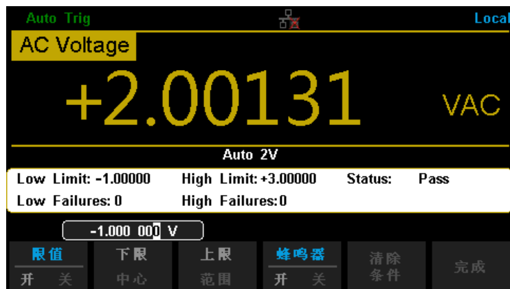
图 3-8 设置下限值
