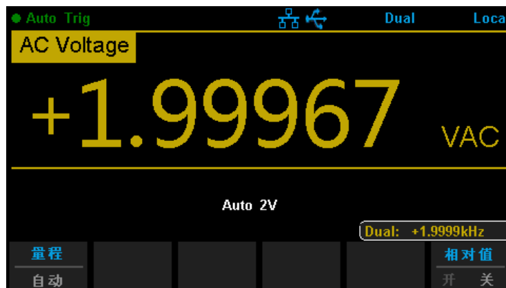
图 2-10 交流电压和频率测量界面
