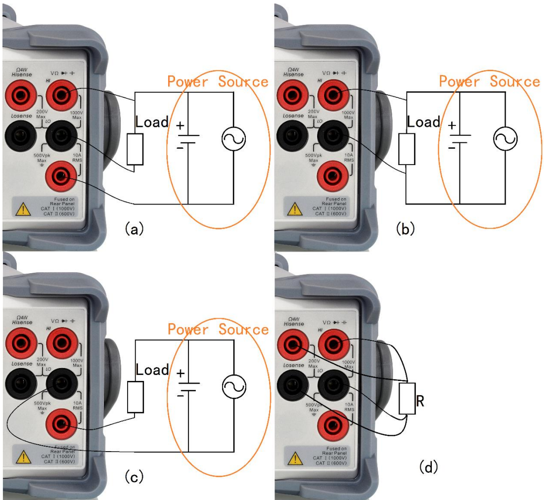
图 2-48 接线示例
