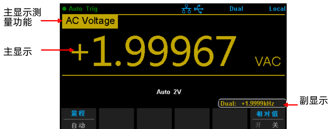
图 1-8 双显用户界面
