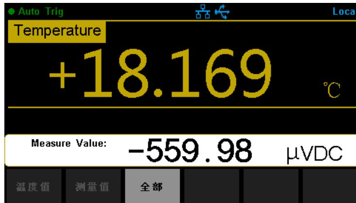
图 2-32 温度测量同时显示对应值和测量值
