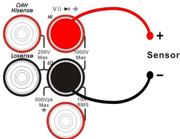
图 2-28 测量温度示意图
