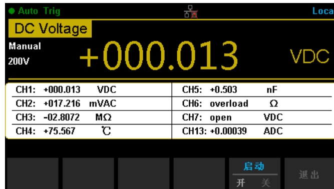
图 2-37 启动扫描后界面
