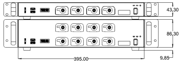
正视图
