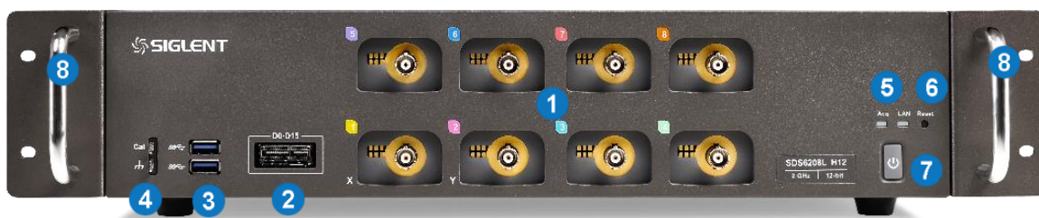
前面板
