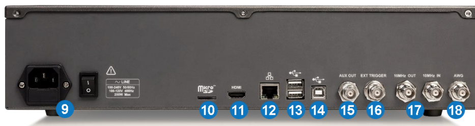
后面板
