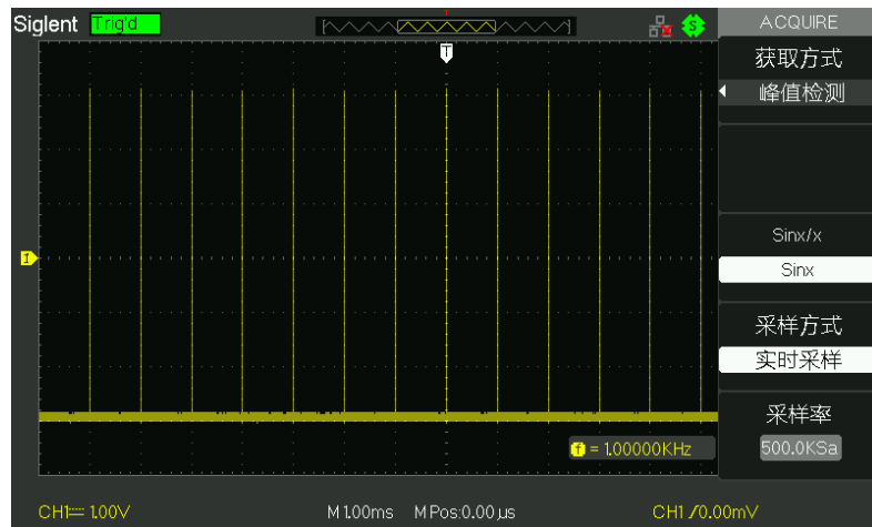
图 2-33 峰值检测模式
