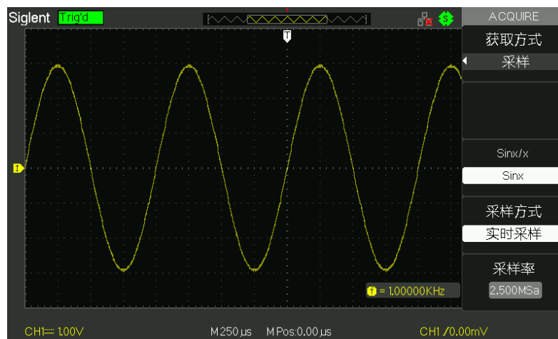
图 2-32 采样模式
