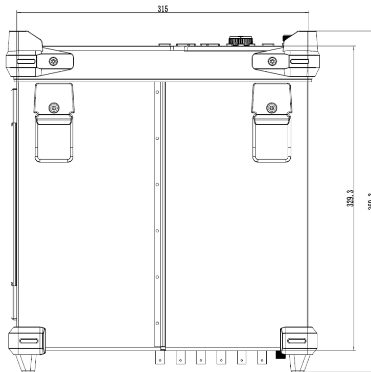
俯视图
