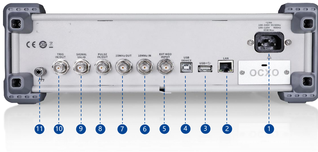
图 1-10 后面板
