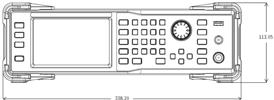
图 1-1 正视图
