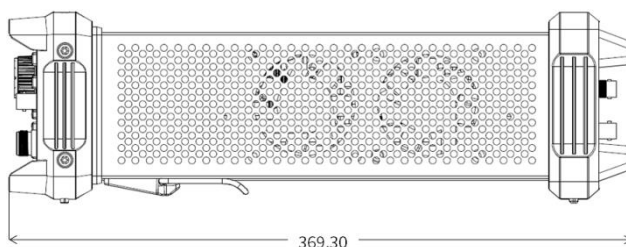
图 1-3 侧视图
