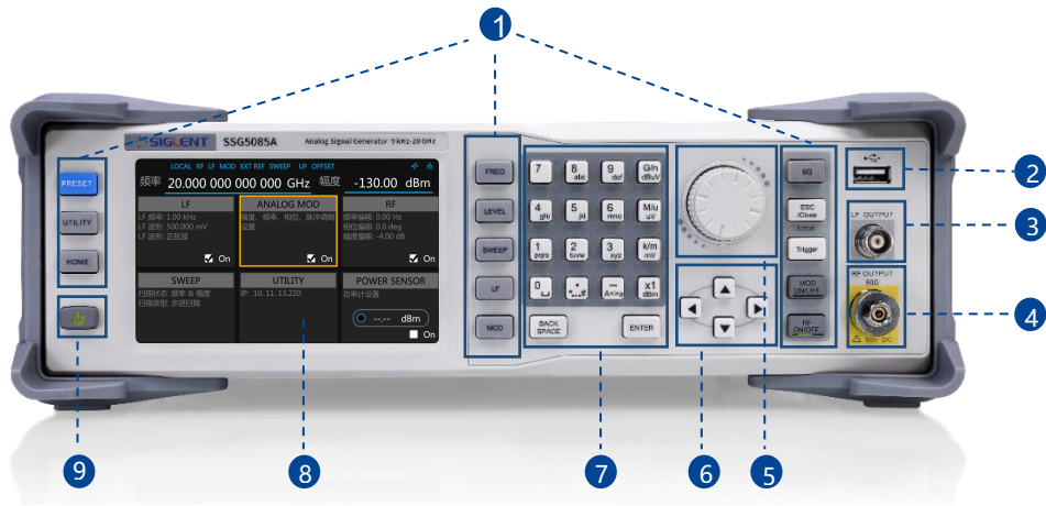
图 1-7 前面板
