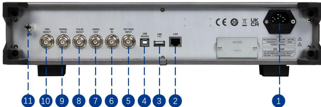
图 6-4 后面板
