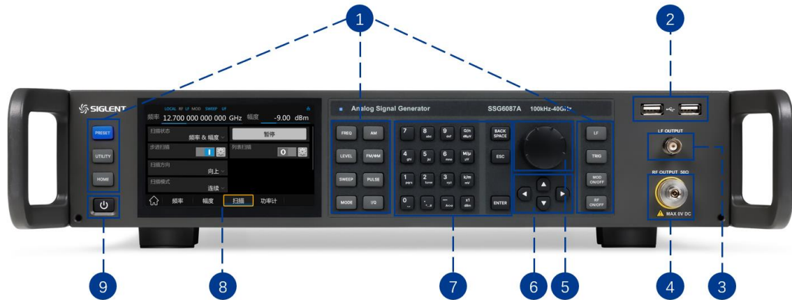
图 6-1 前面板
