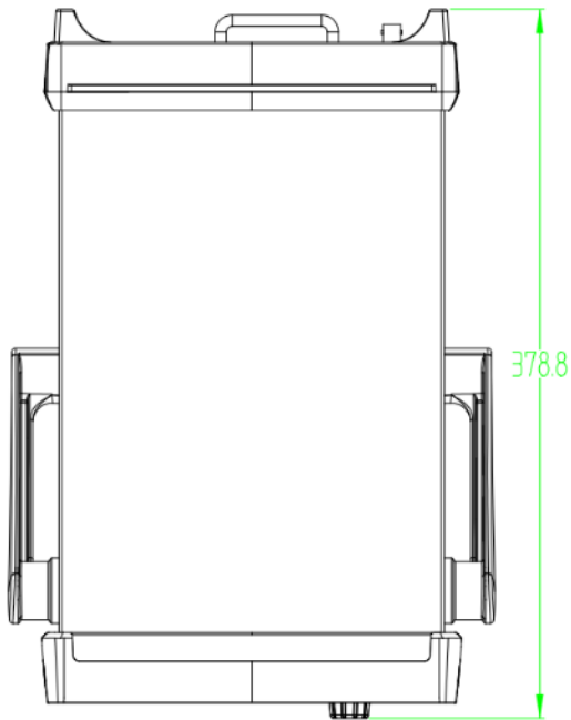
俯视图
