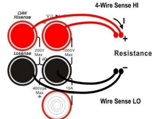
四线电阻测量 (Ω4W)
