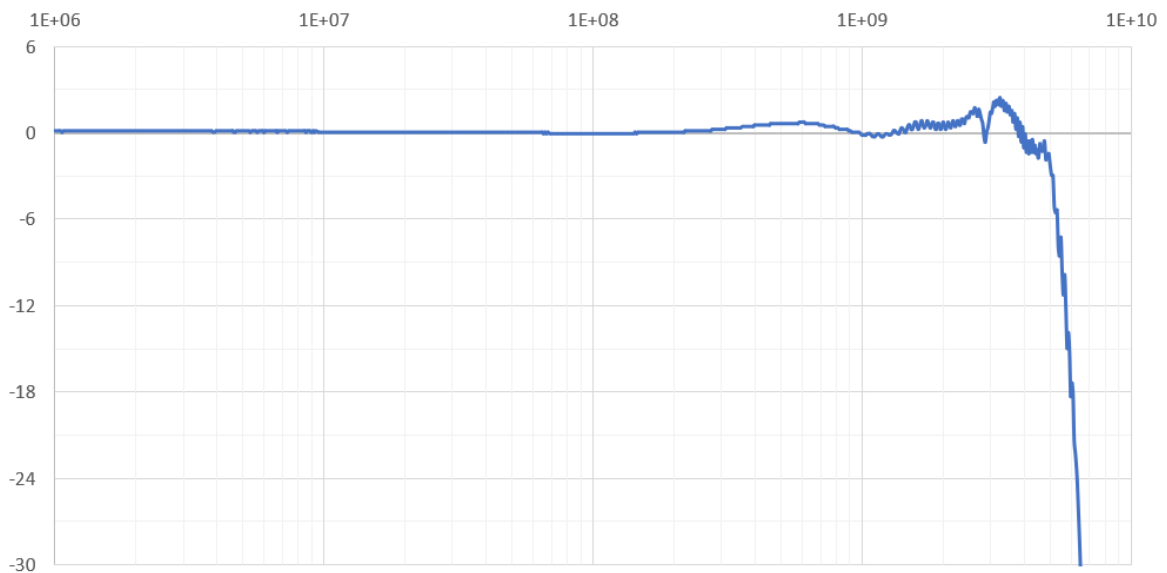
DBT-50 频响曲线（搭配钨钢探针）
