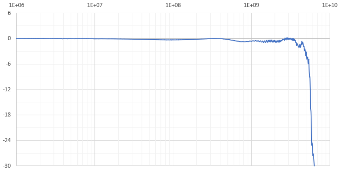
DRP-45 频响曲线
