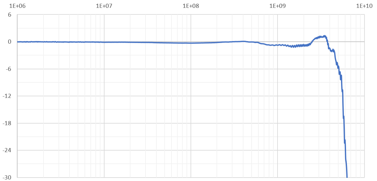
SRP-45 频响曲线
