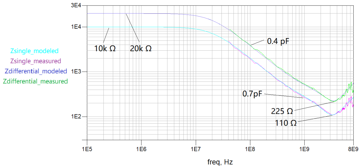
SAP5000D 输入阻抗曲线 (DSI-50 焊接 24.9 Ω 引线电阻)
