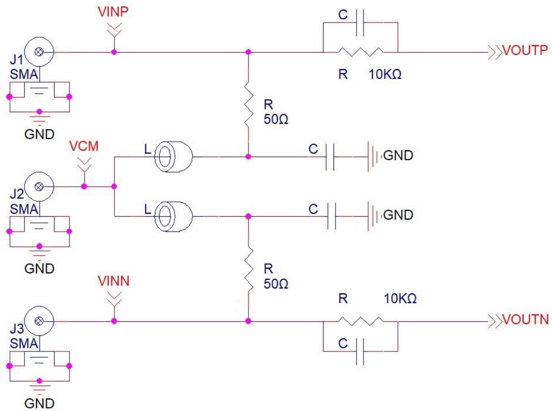
SMA-50 内部原理图
