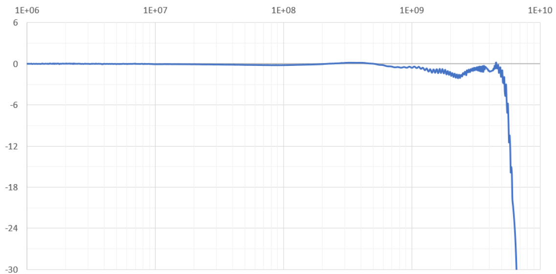
SMA-50 频响曲线
