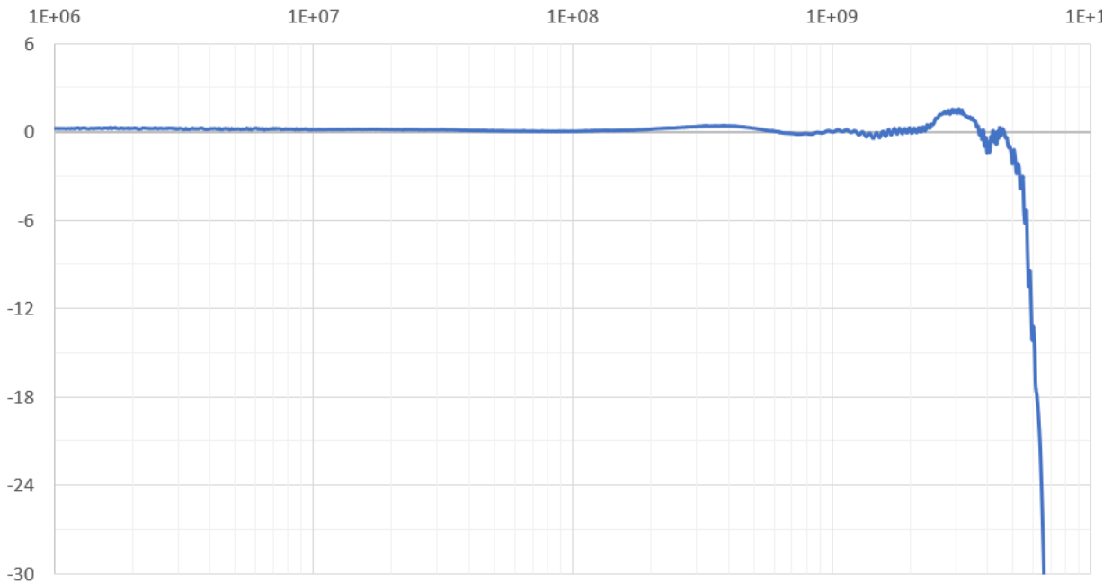
SAP5000D 频率响应曲线 (DSI-50 焊接 24.9 Ω引线电阻)
