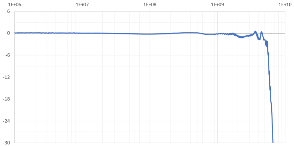
SSI-50 频响曲线（焊接 24.9 R 电阻）
