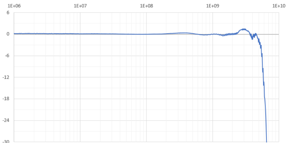
DSI-50 频响曲线 (焊接 24.9 R 电阻)
