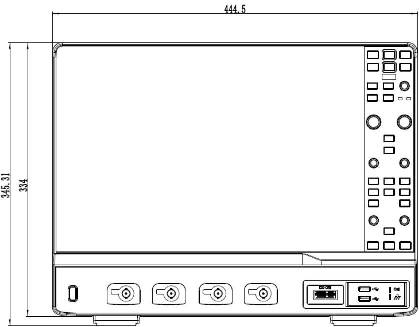
SDS7000A 正视图
