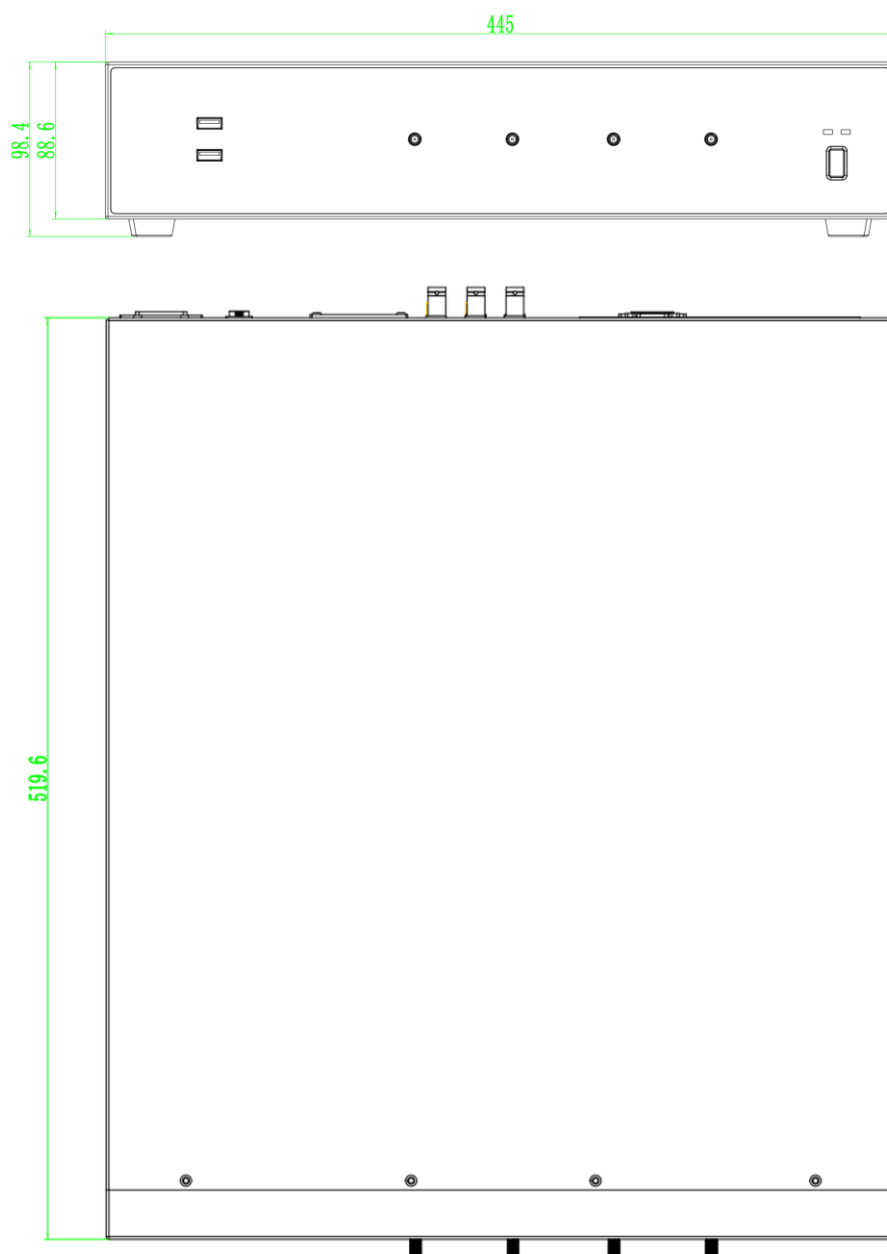
SDS7000L 正视图 & 俯视图
