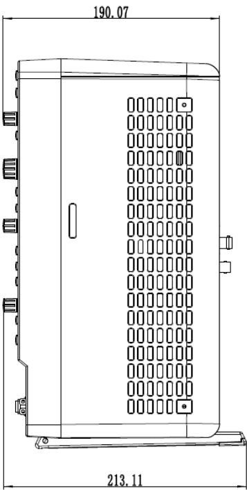
SDS7000A 右视图
