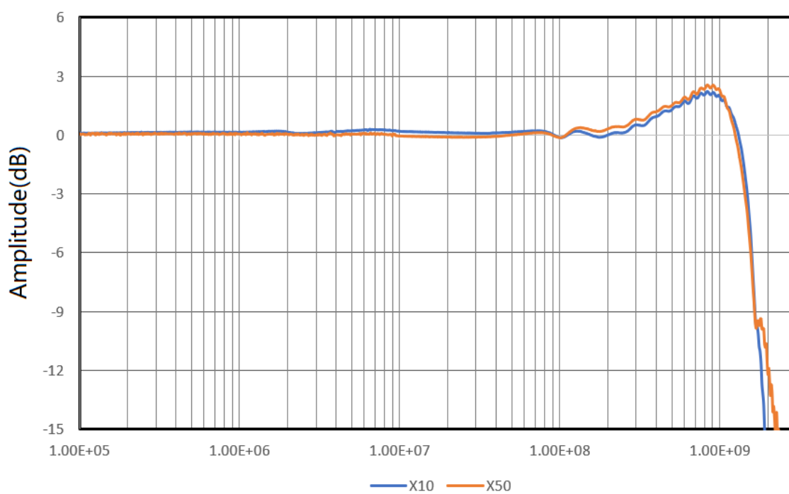
幅频响应
