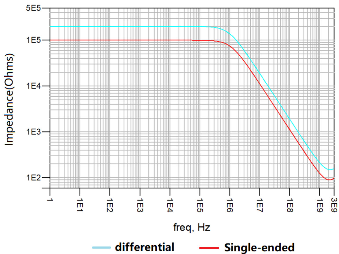
输入阻抗
