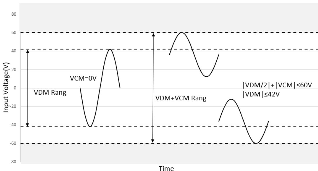
用于差分测量时共模电压和差模电压的要求示意图
