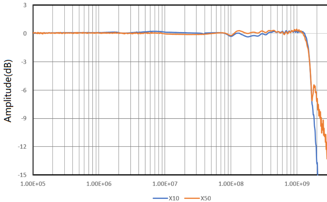
幅频响应
