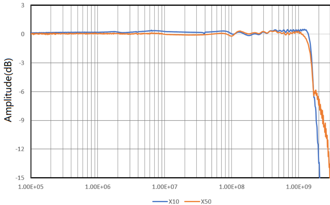
幅频响应
