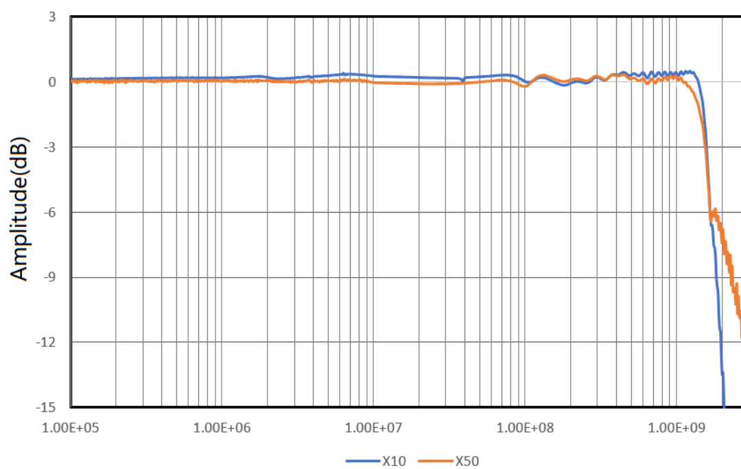
幅频响应
