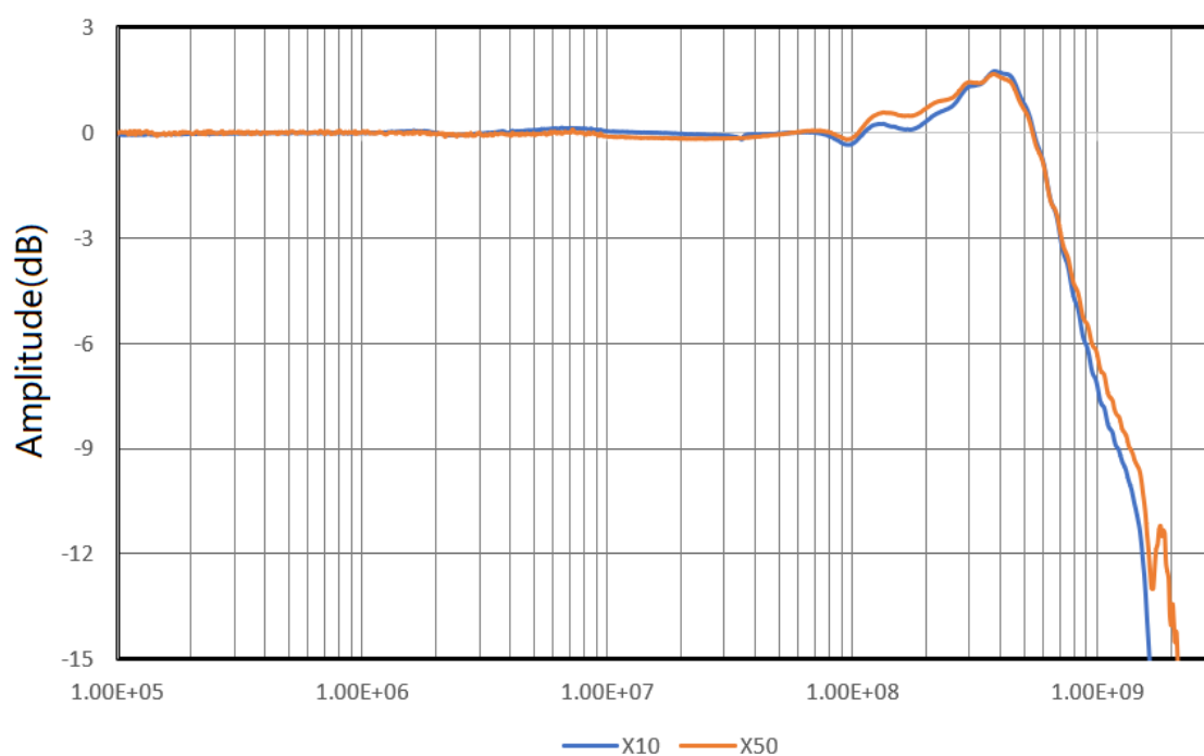
幅频响应
