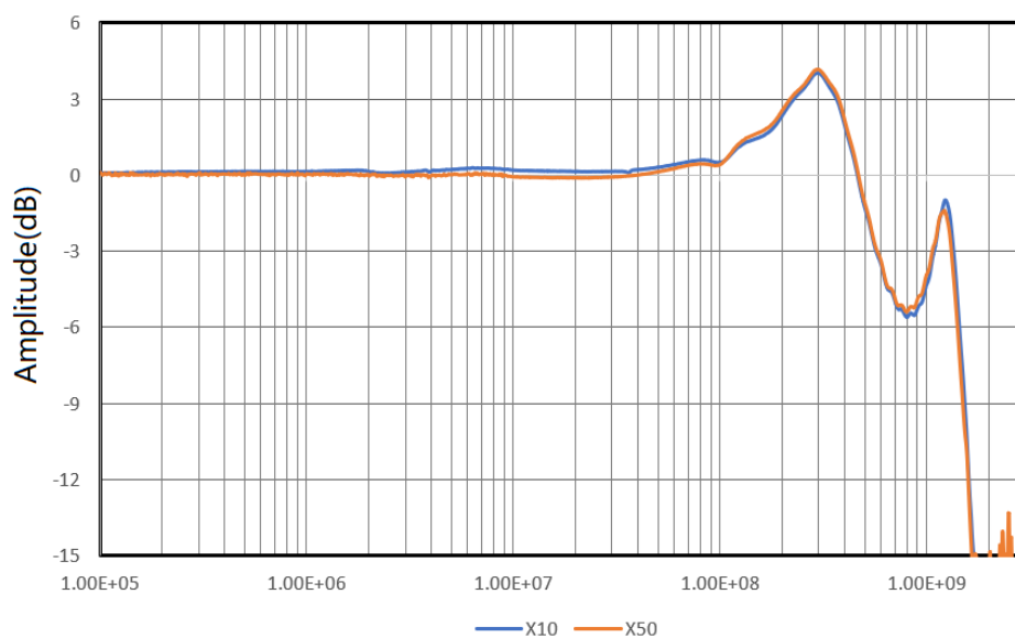
幅频响应
