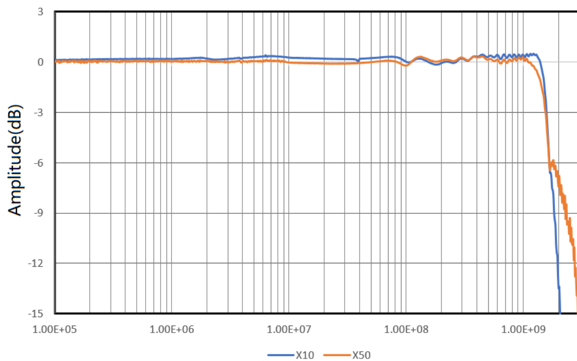
幅频响应
