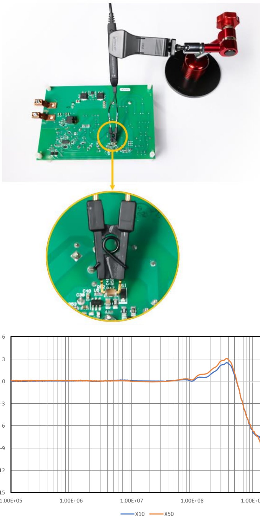
幅频响应
