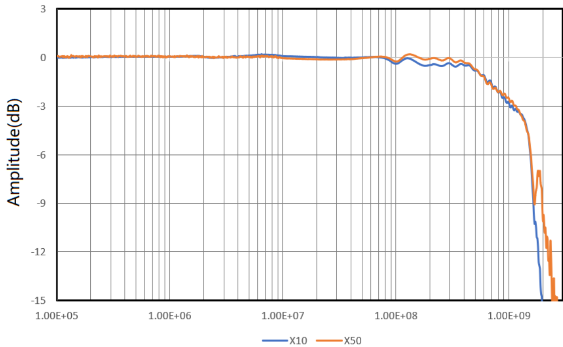
幅频响应
