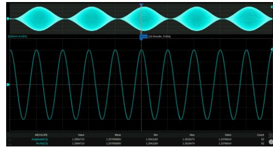
100%调制深度时域图
