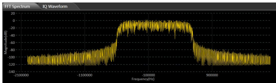
图 9-7 EasyIQ 波形频谱图
