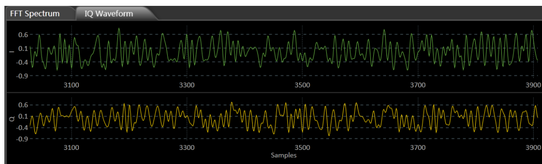
图 9-8 EasyIQ 时域波形图
