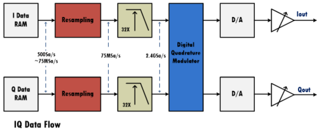
图 9-2 SDG6000X 中的 I/Q 信号流图
