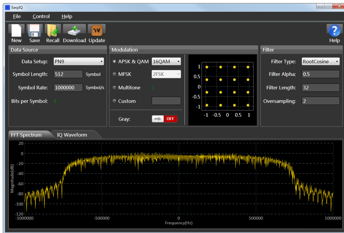
图 9-3 EasyIQ 界面
