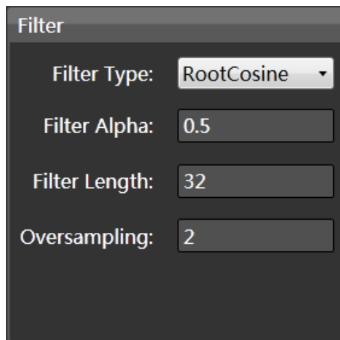
图 9-6 EasyIQ 滤波器界面
