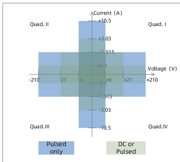
最大电压和最大电流工作范围
