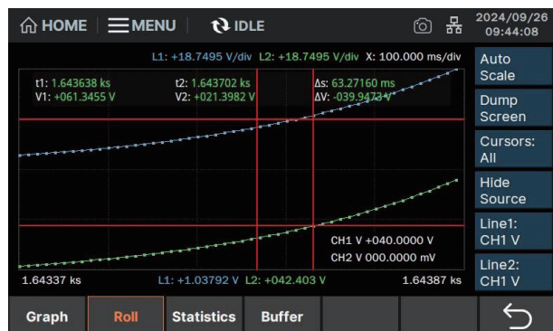
Roll 视图
