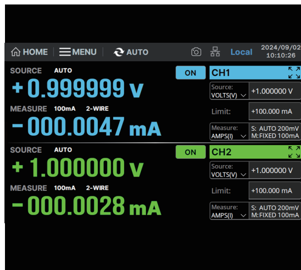
双通道显示
