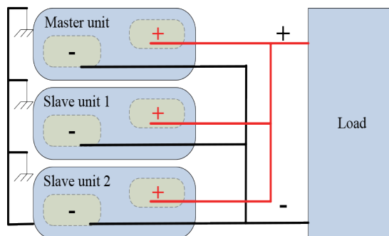
并联模式
