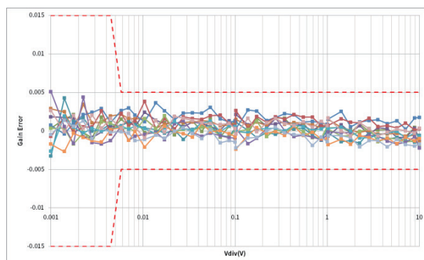
0.5% 的直流增益精度
