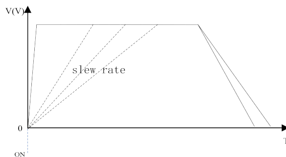
可调输出电压电流上升 / 下降斜率
