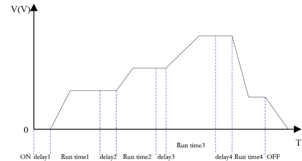
List 模式
