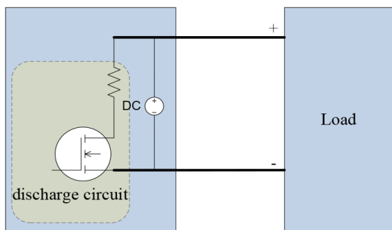
泄放电路
